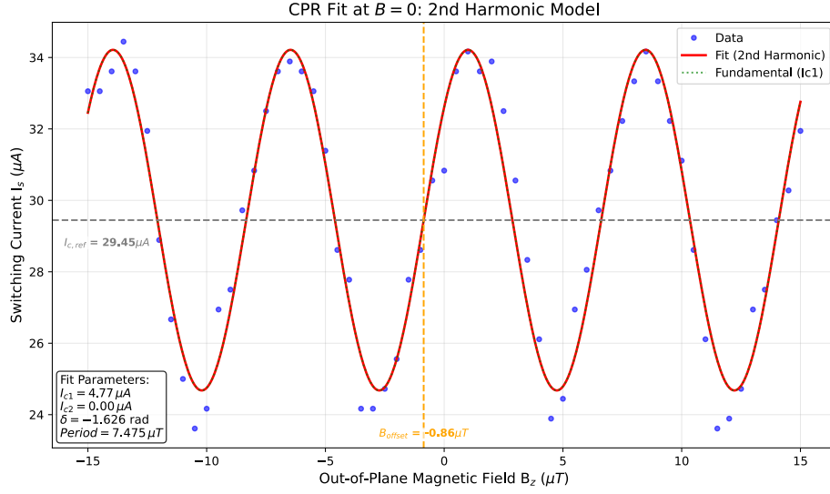
圖 24 使用二階諧波相位差可調模型擬合典型 PtTe 2 約瑟夫森接面的電流相位關係特性曲線
