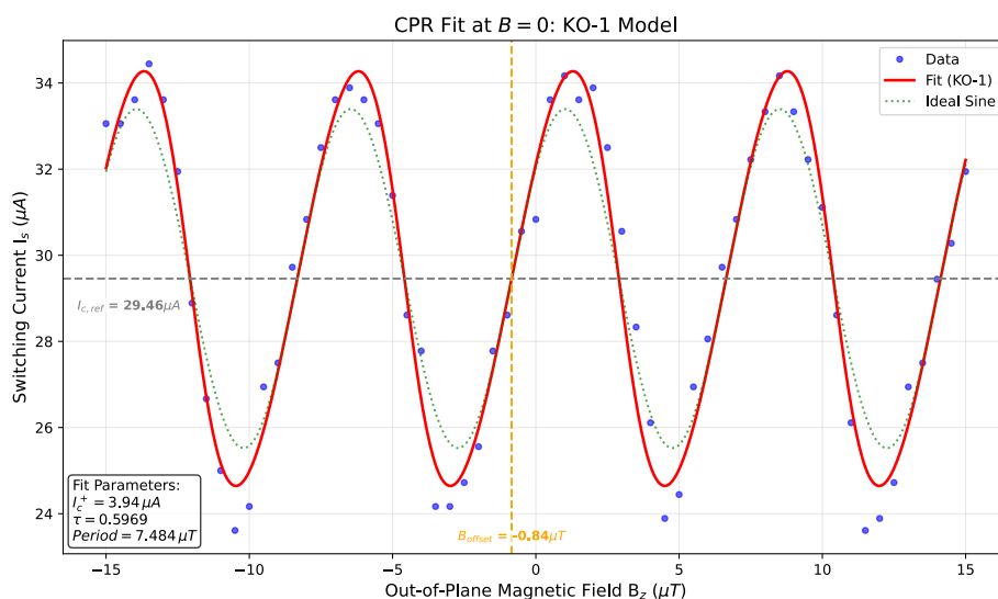
圖 23 使用 Kulik-Omelyanchuk 模型擬合典型 \text{PtTe}_2 約瑟夫森接面的電流相位關係特性曲線
