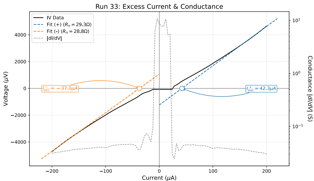
圖 8 樣品 004-1 的多重安德烈夫反射特性展示
