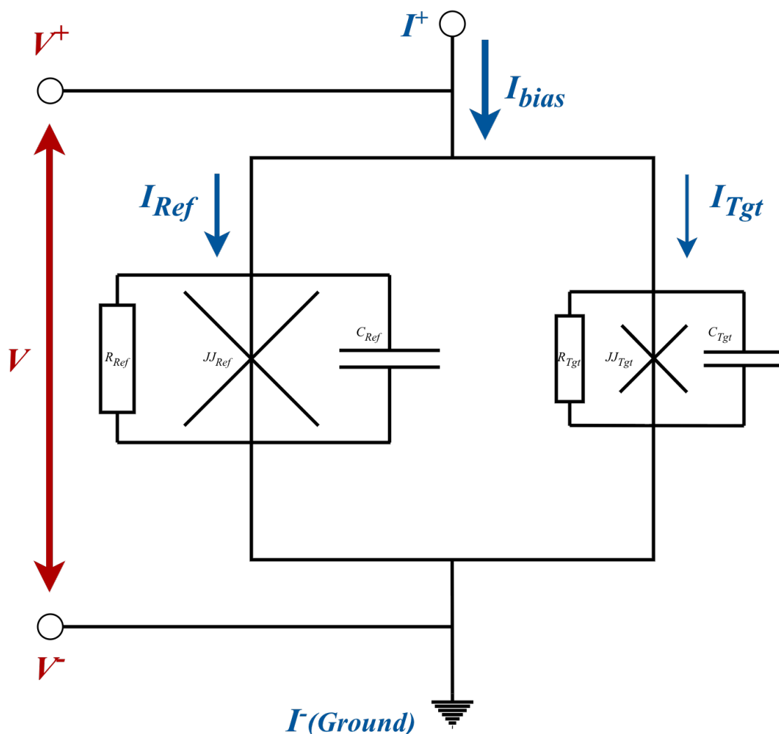
圖 1 DC SQUID 示意圖：兩個約瑟夫森接面（以叉號表示）並聯於一個電感為 L 的超導環上。偏置電流 (bias current) I 分流通過兩個臂，外加磁通量 \Phi_{ext} 穿過環路。
