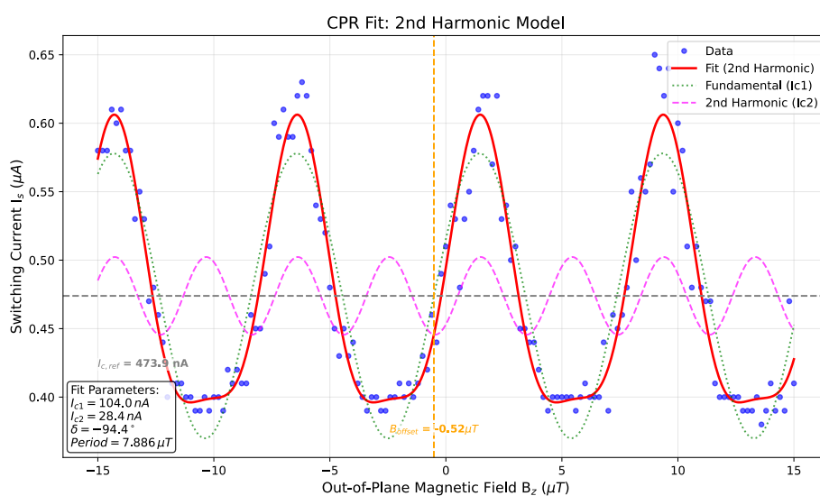
圖 25 樣品 003-2 在面內磁場強度為 180 mT，角度為 297.4^\circ 的二階諧波相位差可調模型擬合結果
