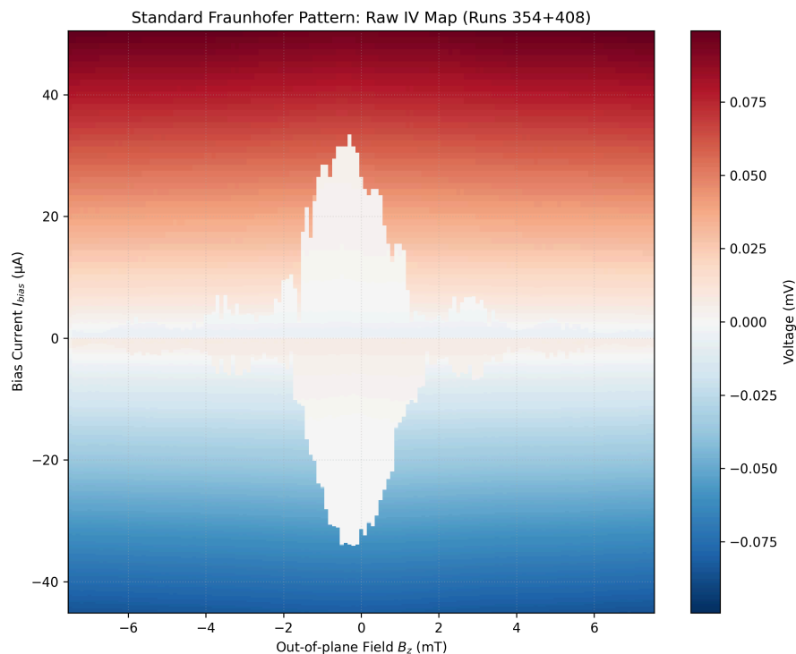
圖 11 夫朗和費干涉圖樣的原始量測數據熱圖 ( V vs I, B_z )。
