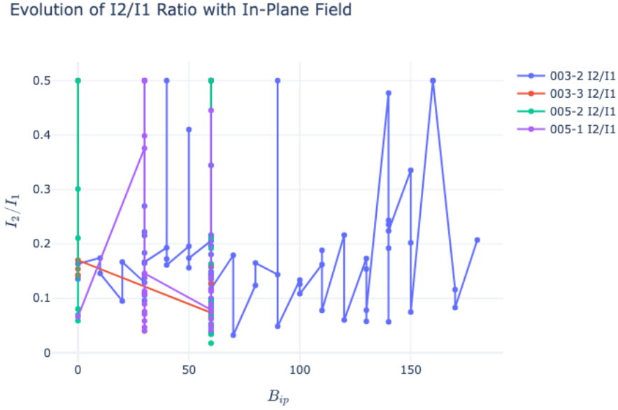
圖 29 二階諧波分量 ( \frac{I_2}{I_1} ) 隨面內磁場的演化。
