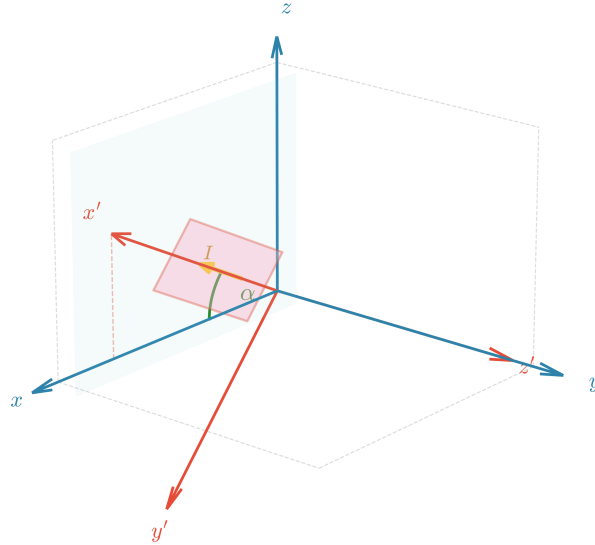
圖 9 實驗室座標系 (X, Y, Z) (藍色) 與樣品座標系 (X', Y', Z') (紅色) 之幾何關係。
