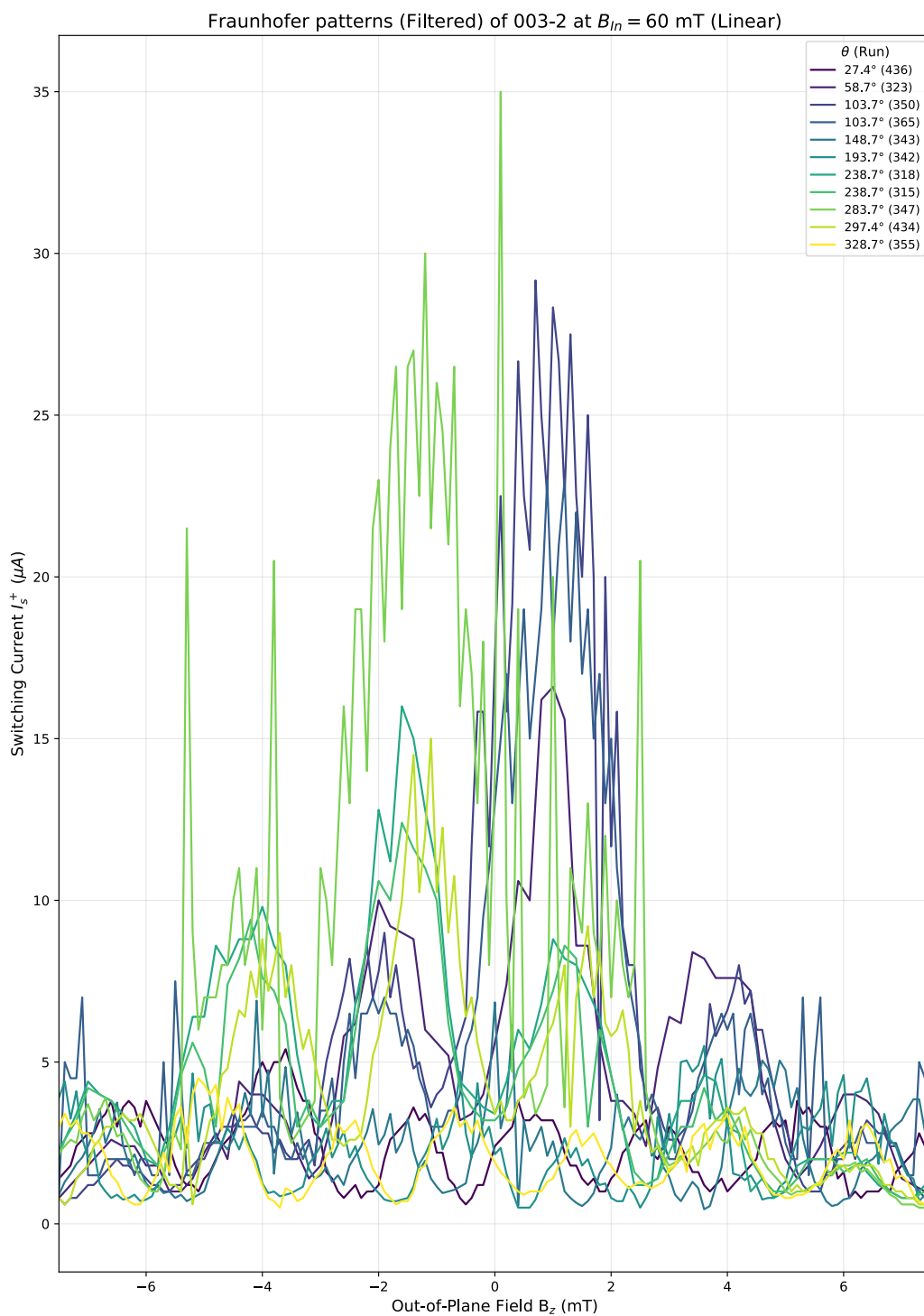
圖 13 樣品 003-2 在面內磁場 B_{\text{In-Plane}} 固定在 60 mT 時，夫朗和費圖樣隨角度 \theta 的演化。
