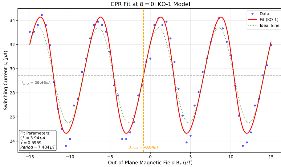
圖 23 使用 KO-1 模型擬合典型 PtTe 2 約瑟夫森接面的電流相位關係特性曲線 使用 KO-1 模型擬合典型 PtTe 2 約瑟夫森接面的電流相位關係特性曲線。
