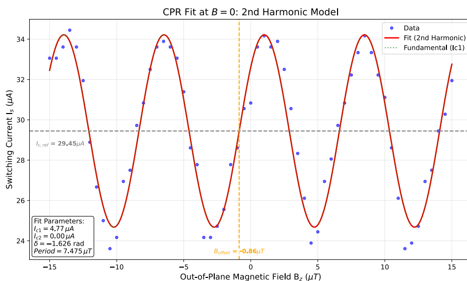
圖 24 使用二階諧波相位差可調模型擬合典型 \text{PtTe}_2 約瑟夫森接面的電流相位關係特性曲線
