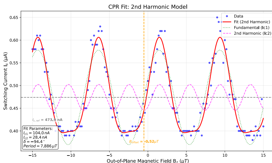
圖 25 樣品 003-2 在面內磁場強度為 180 mT，角度為 297.4° 的二階諧波相位差可調模型擬合結果
