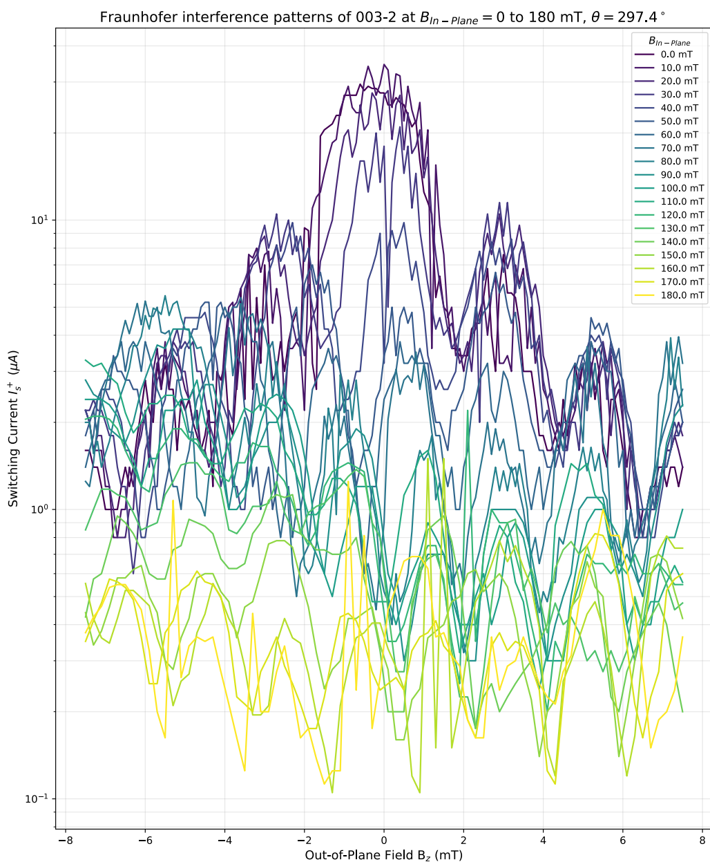
圖 17 樣品 003-2 在面內磁場角度 \theta 固定在 297.4^\circ 時，夫朗和費圖樣隨磁場強度
