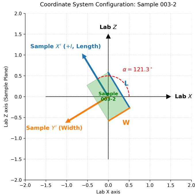
圖 10 Sample 003-2 的座標系配置示意圖。樣品位於實驗室 X-Z 平面，逆時針旋轉角度 \alpha = 121.3^\circ 。綠色矩形代表樣品，藍色箭頭指示沿長軸的電流方向 ( x' axis)。
