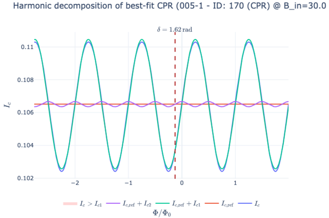
圖 26 重構的 PtTe 2 接面電流-相位關係 (Sample 005-1, Run 170)。實驗數據與擬合結果顯示了顯著的非純正弦特徵。
