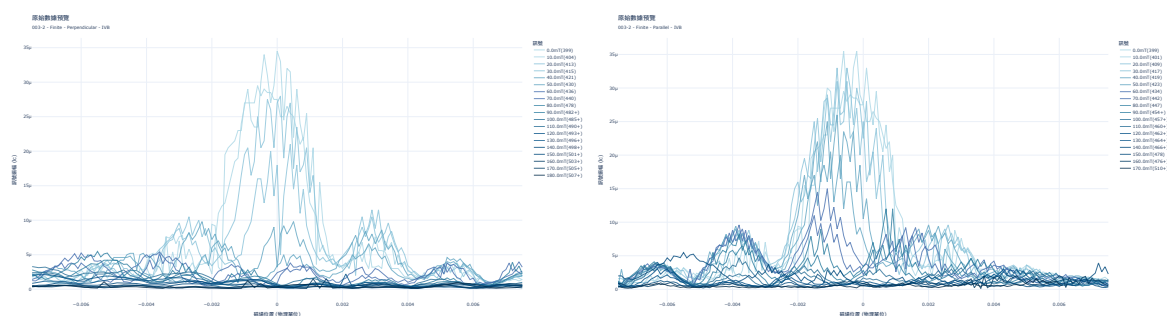
圖 19 垂直/平行電流方向磁場下夫朗和費圖樣的演化
