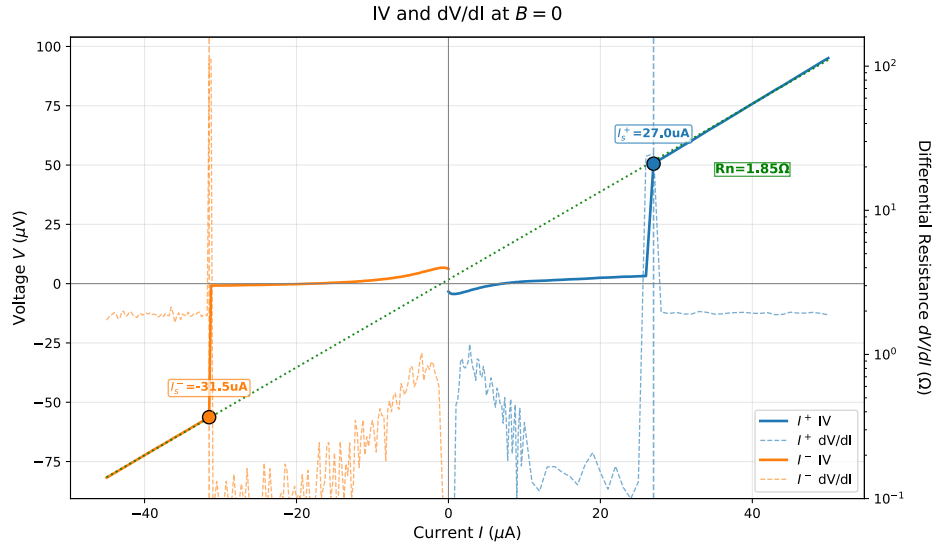
圖 7 典型 \text{PtTe}_2 約瑟夫森接面的正負向切換電流 I - V 特性曲線
