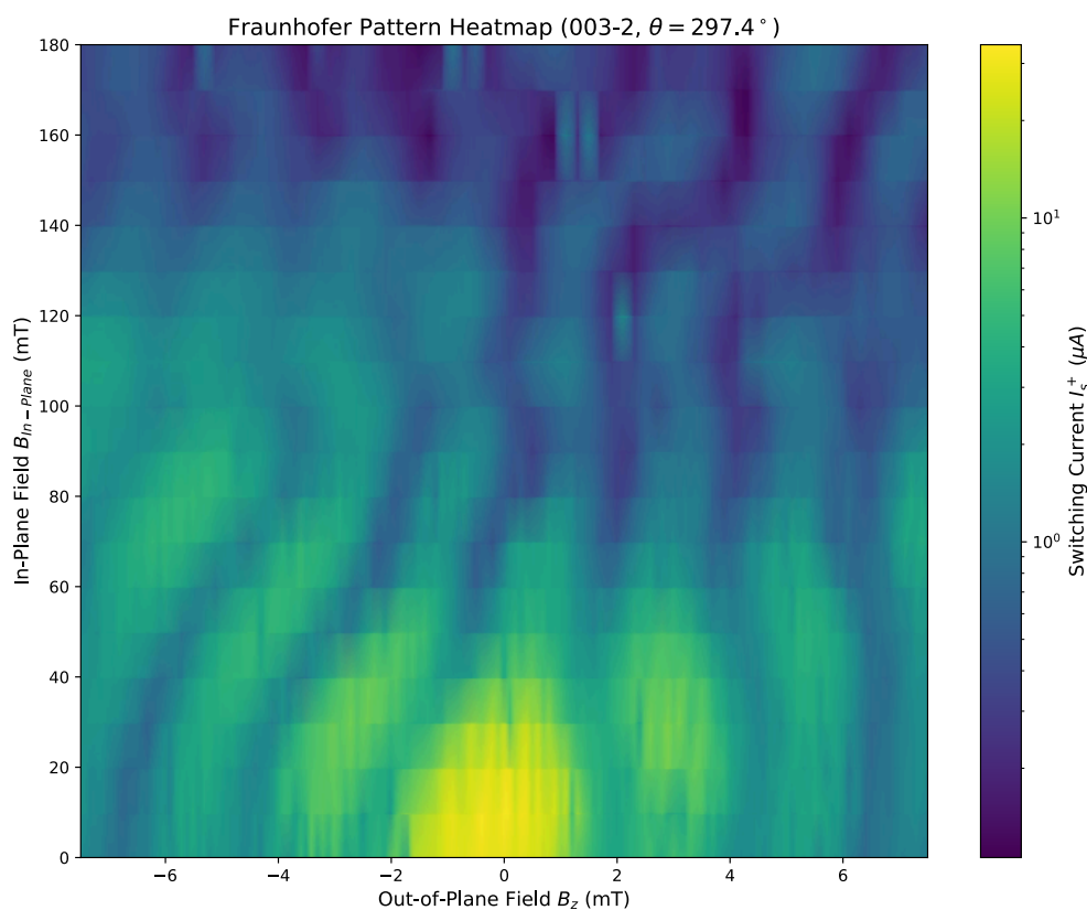
圖 18 樣品 003-2 在面內磁場角度 \theta 固定在 297.4^\circ 時，夫朗和費圖樣隨磁場強度 B_{\text{In-Plane}} 的演化熱圖。
