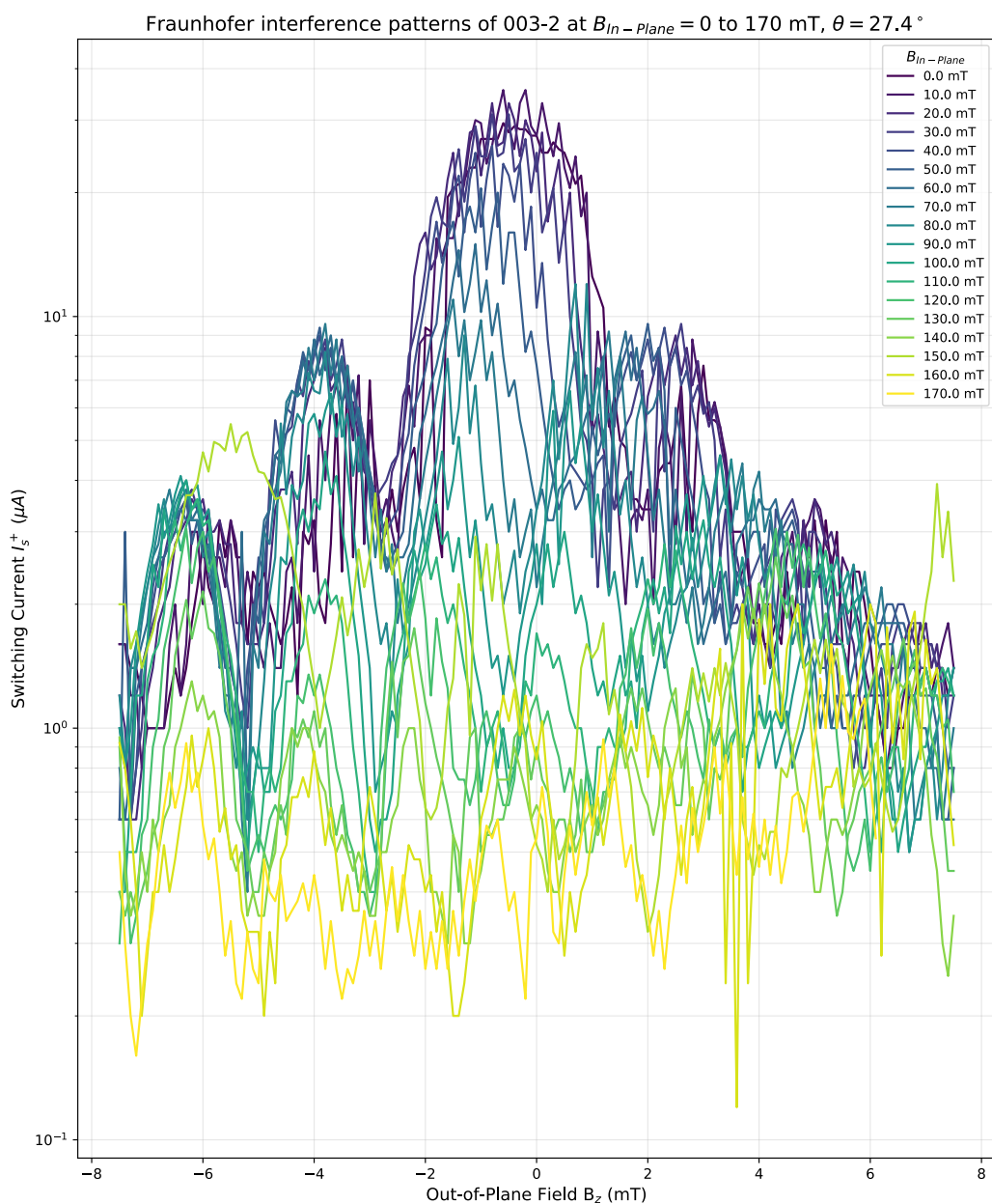
圖 15 樣品 003-2 在面內磁場角度 \theta 固定在 27.4^\circ 時，夫朗和費圖樣隨磁場強度 B_{In-Plane} 的演化。
