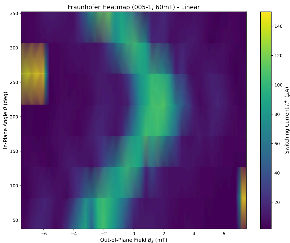
圖 14 樣品 005-1 在面內磁場 B_{\text{In-Plane}} 固定在 60 mT 時，夫朗和費圖樣隨角度 \theta 的演化熱圖。
