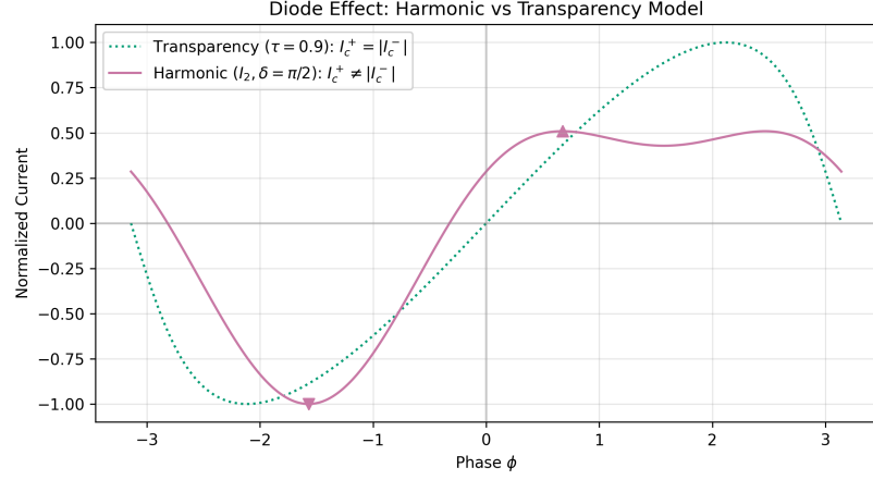
圖 22 透明度模型與諧波模型的比較。標準透明度模型 (綠線) 雖然能產生偏斜的波形，但仍保持 I_c^+ = |I_c^-| 的對稱性。含有相位偏移的諧波模型 (紫線) 則能自然描述 I_c^+ \neq |I_c^-| 的約瑟夫森二極體效應。
