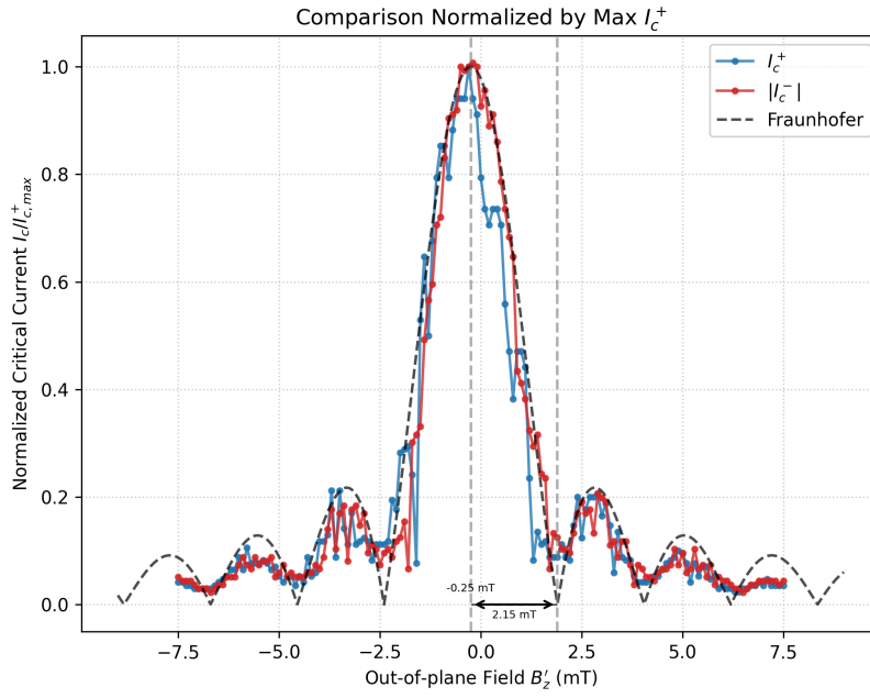
圖 12 正規化切換電流 ( I_s ) 隨面外磁場 ( B_{z'} ) 的變化。
