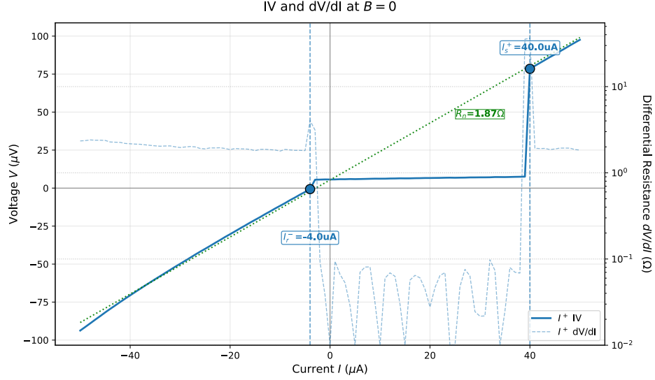
圖 6 典型 \text{PtTe}_2 約瑟夫森接面的負向重捕電流及正負向切換電流 I - V 特性曲線
