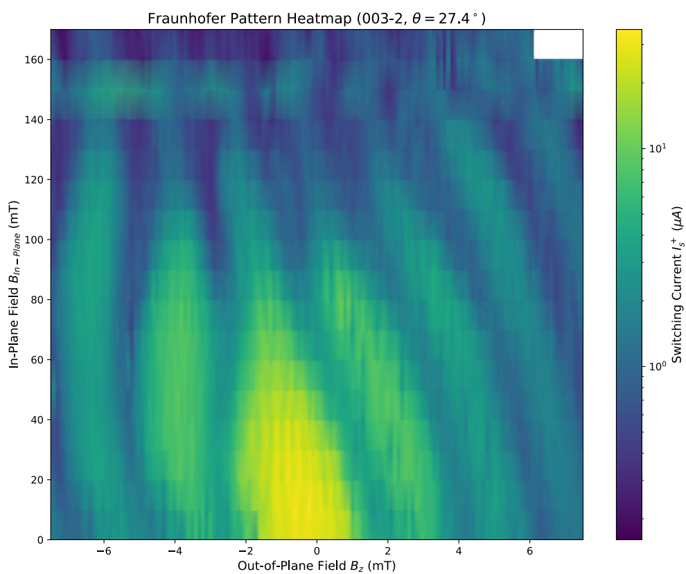
圖 16 樣品 003-2 在面內磁場角度 \theta 固定在 27.4^\circ 時，夫朗和費圖樣隨磁場強度 B_{\text{In-Plane}} 的演化熱圖。
