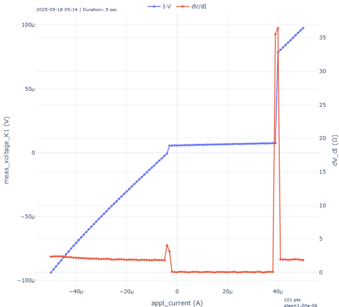
圖 6 典型 PtTe 2 約瑟夫森接面的 I-V 特性曲線
