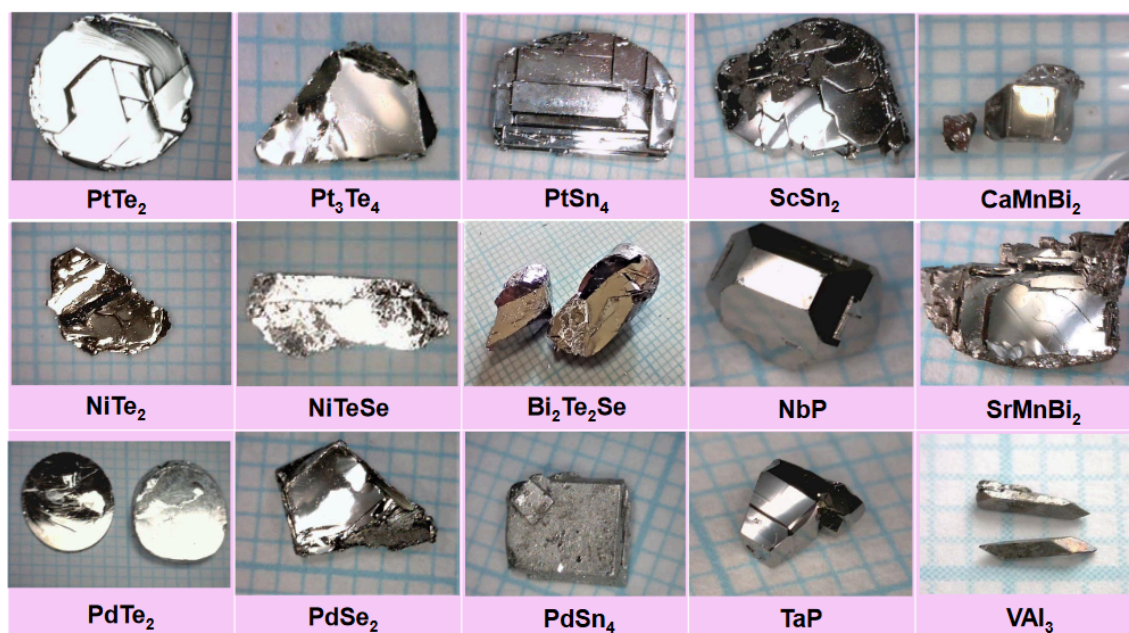
圖 5 拓樸材料晶體。Ref.[5]
