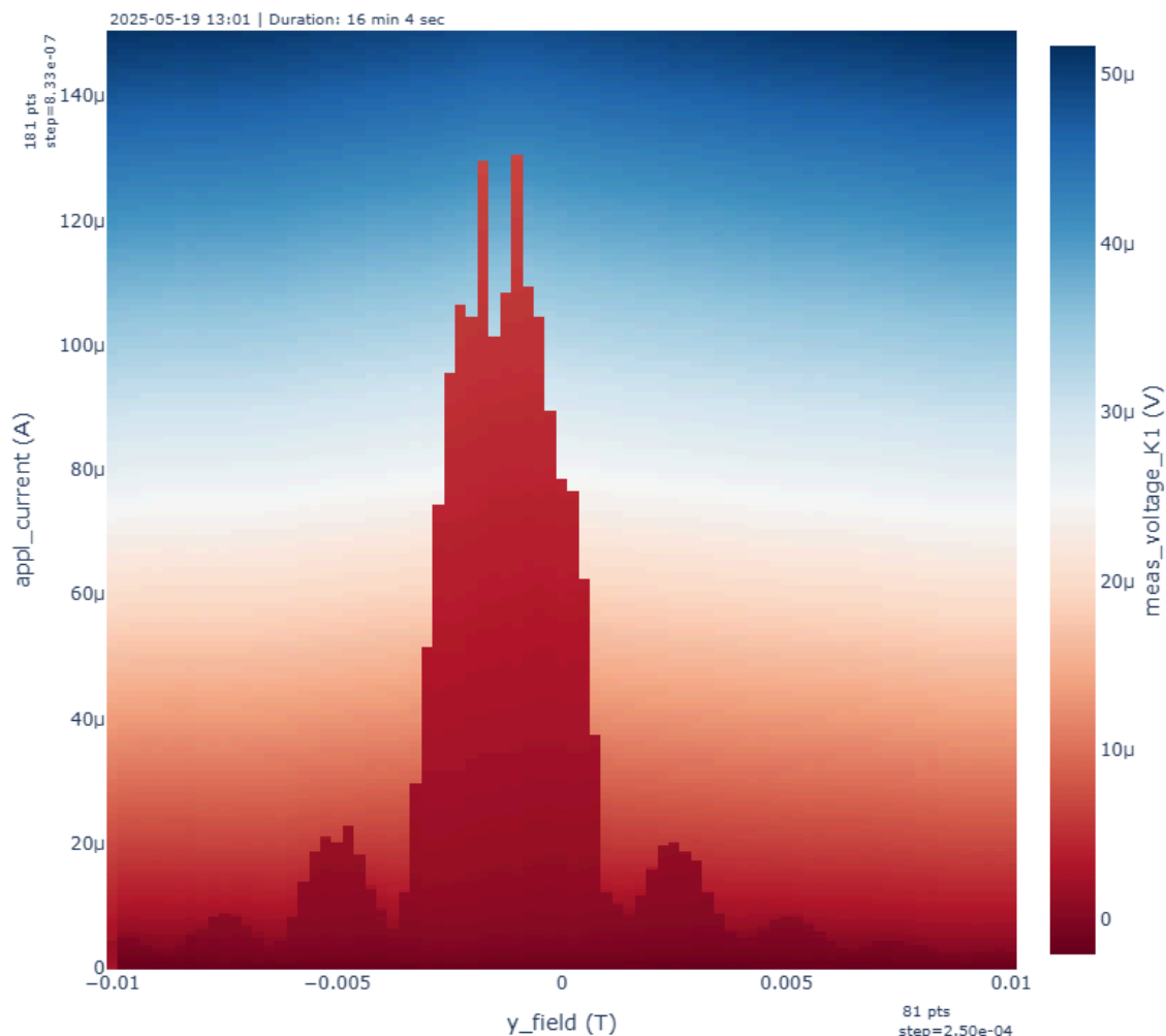
圖 9 標準夫朗和費干涉圖樣 ( B_{\parallel} = 0 )
