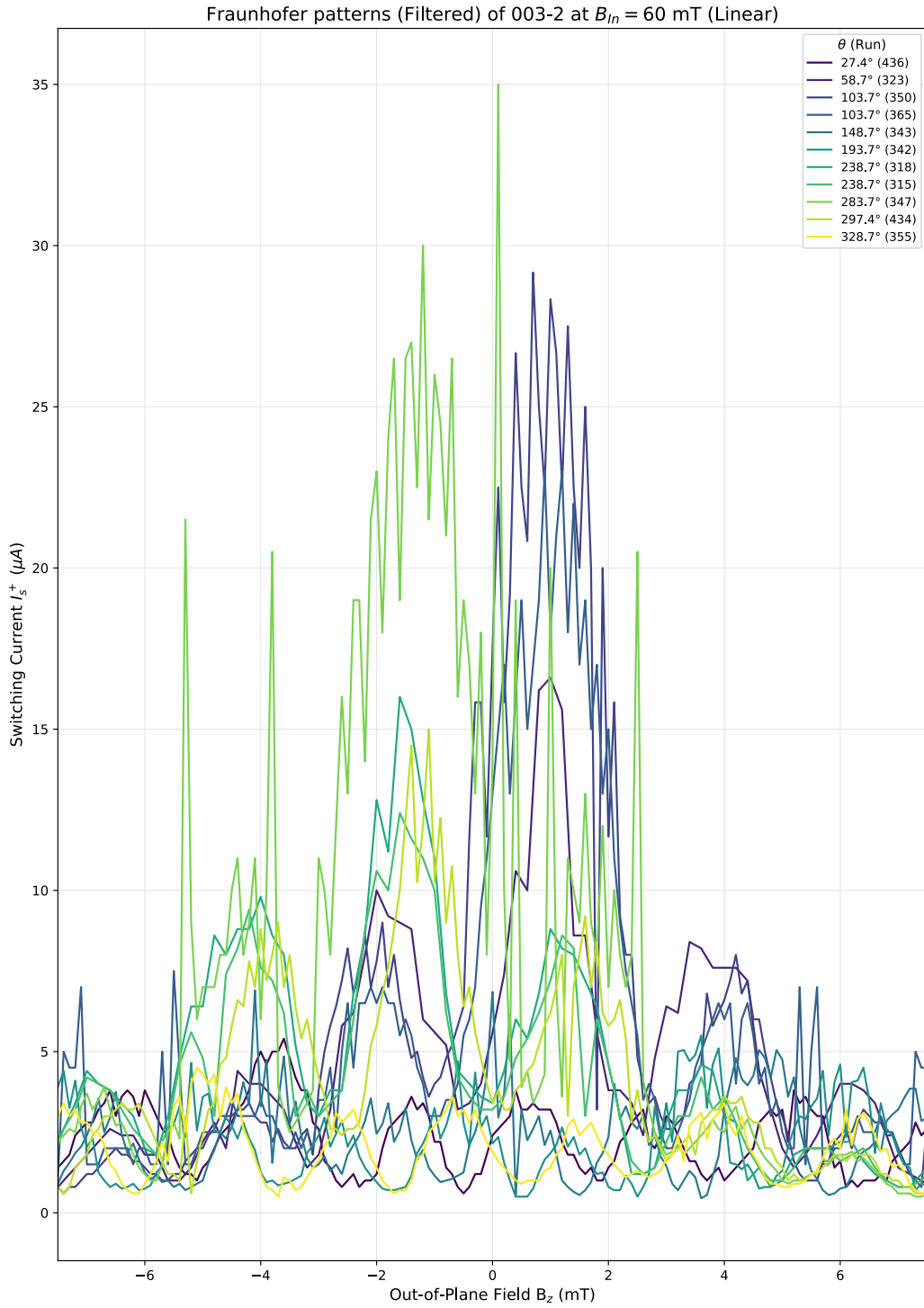
圖 13 樣品 003-2 在面內磁場 B_{In-Plane} 固定在 60 mT 時，夫朗和費圖樣隨角度 \theta 的演化。
