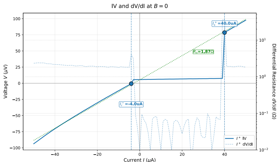
圖 6 樣品 003-2 之負向重捕電流及正負向切換電流 I-V 特性曲線
