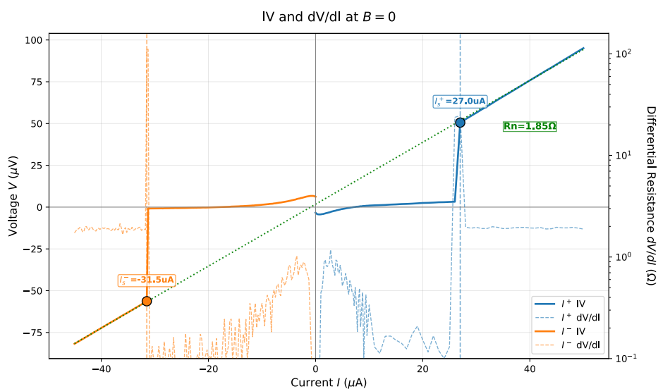
圖 7 樣品 003-2 之正負向切換電流 I-V 特性曲線
