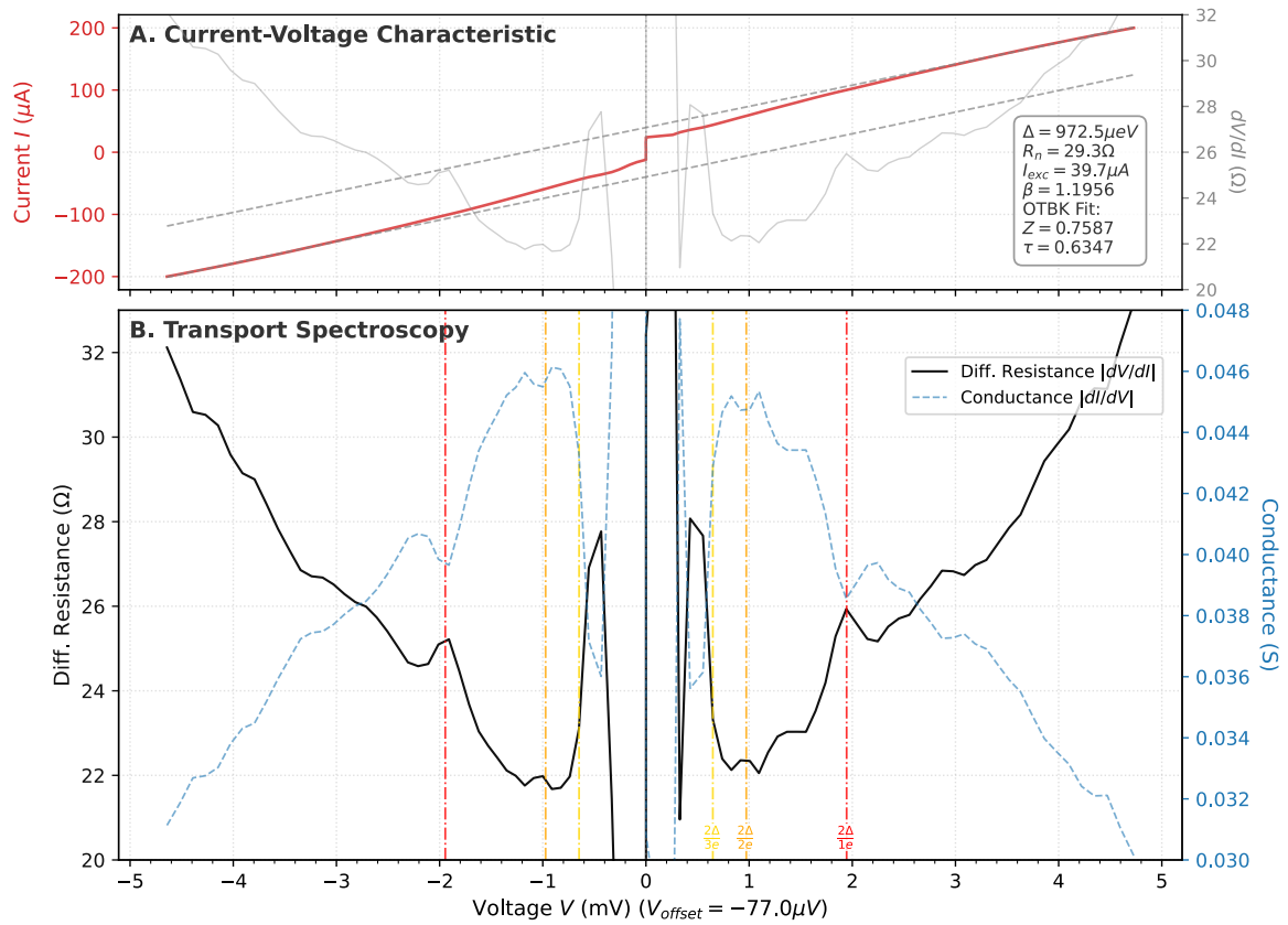
圖 8 PtTe 2 約瑟夫森接面的直流傳輸特性與多重安德烈夫反射 (MAR)。(a) 在基溫 ( T \approx 40, \text{mK} ) 下量測之電流-電壓 ( I - V ) 特性曲線。接面展現出清晰的超電流分支 (Supercurrent branch)，其切換電流 (Switching current) I_c \approx 24, \mu\text{A} 。高偏壓處的過剩電流 ( I_{\text{exc}} ，灰色虛線所示) 顯示該接面具有中透明度的介面特性。(b) 微分電阻 ( dV/dI ) 隨量測電壓 V 的變化曲線。頻譜中展現一系列對應於次諧波能隙結構 (Sub-harmonic gap structures) 的電阻峰。垂直虛線標示了 MAR 特徵峰的理論預期位置 ( V_n = 2\Delta / ne ，其中 n = 1, 2, 3 )，由此推算出超導能隙 \Delta \approx 0.9725 \text{ meV} 。並以 OBTK 模型的最佳擬合曲線，提取出的介面阻抗參數 Z \approx 0.7587 與穿透率 \tau \approx 0.6347 並以 \beta \approx
