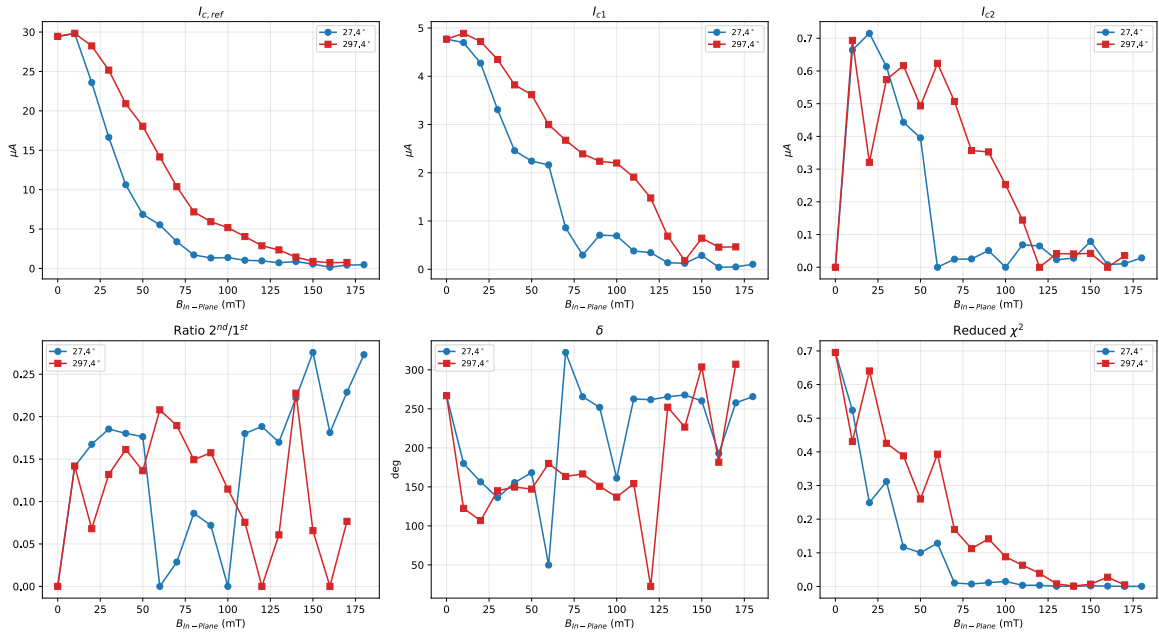
圖 27 CPR 擬合參數隨面內磁場的演化。
