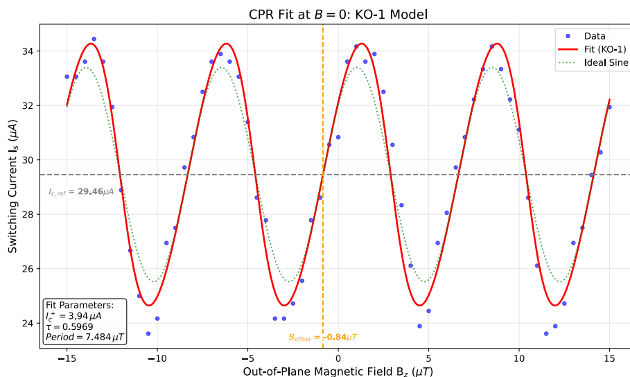
圖 23 使用 Kulik-Omelyanchuk 模型擬合典型 PtTe 2 約瑟夫森接面的電流相位關係特性曲線
