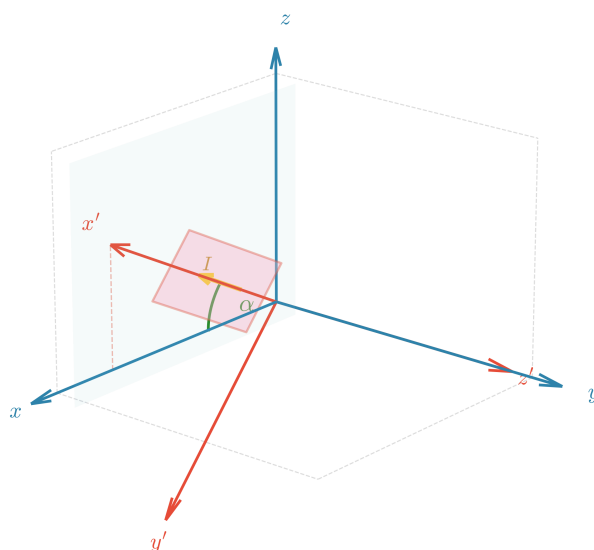
圖 9 實驗室座標系 ( X, Y, Z ) (藍色) 與樣品座標系 ( X', Y', Z' ) (紅色) 之幾何關係。樣品平面 (粉色矩形) 位於 X - Z 平面內，電流方向 X' 與 X 軸夾角為 \alpha 。
