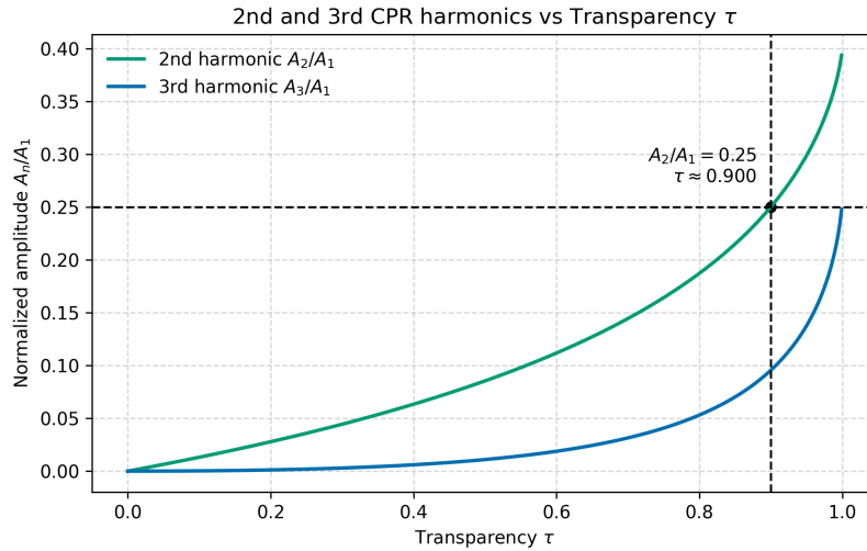
圖 16 二階與三階諧波分量隨透明度 \tau 的變化。為了產生 \frac{I_2}{I_1} = 0.25 的二階分量，透明度必須高達 \tau \approx 0.90 。
