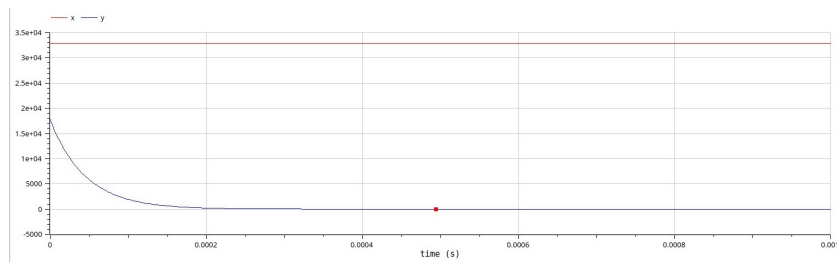
Рис. 4.5: Модель боевых действий с участием регулярных войск и партизанских отрядов
