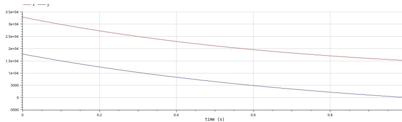
Рис. 4.2: Модель боевых действий между регулярными войсками
