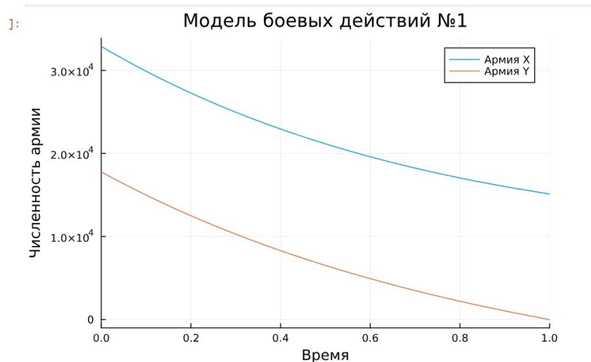
Рис. 4.1: Модель боевых действий между регулярными войсками
