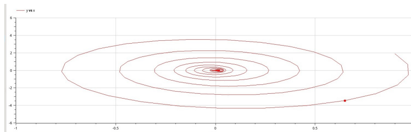
Рис. 4.12: Фазовый портрет колебаний гармонического осциллятора с затуханием и под действием внешней силы. OpenModelica
