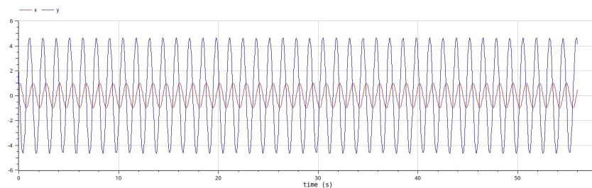
Рис. 4.3: Колебания гармонического осциллятора без затуханий и без действий внешней силы. OpenModelica
