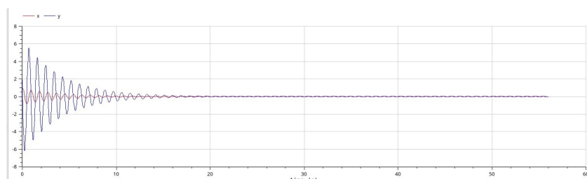
Рис. 4.7: Колебания гармонического осциллятора с затуханием и без действий внешней силы. OpenModelica
