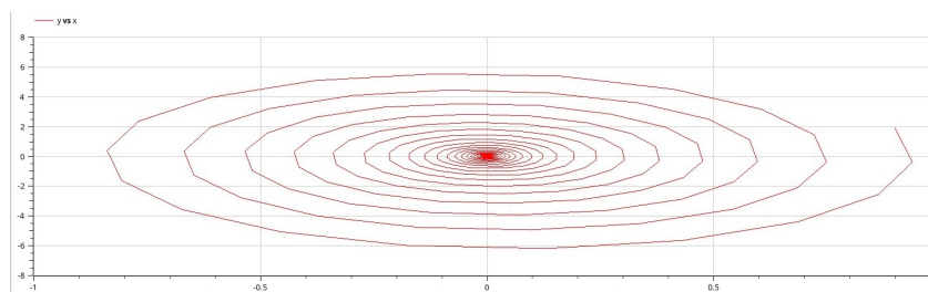
Рис. 4.8: Фазовый портрет колебаний гармонического осциллятора с затуханием и без действий внешней силы. OpenModelica
