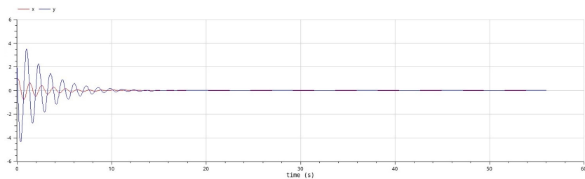
Рис. 4.11: Колебания гармонического осциллятора с затуханием и под действием внешней силы. OpenModelica
