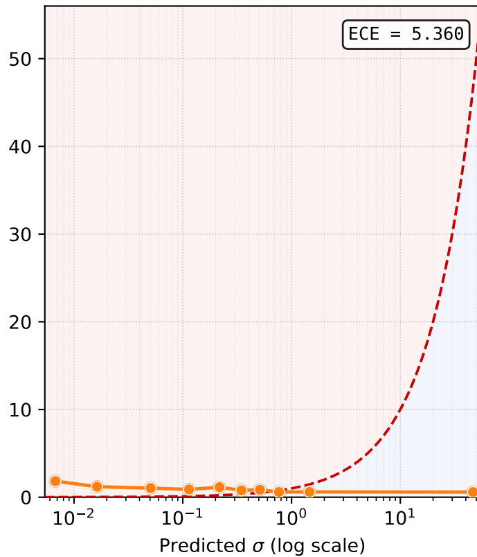
Vanilla
