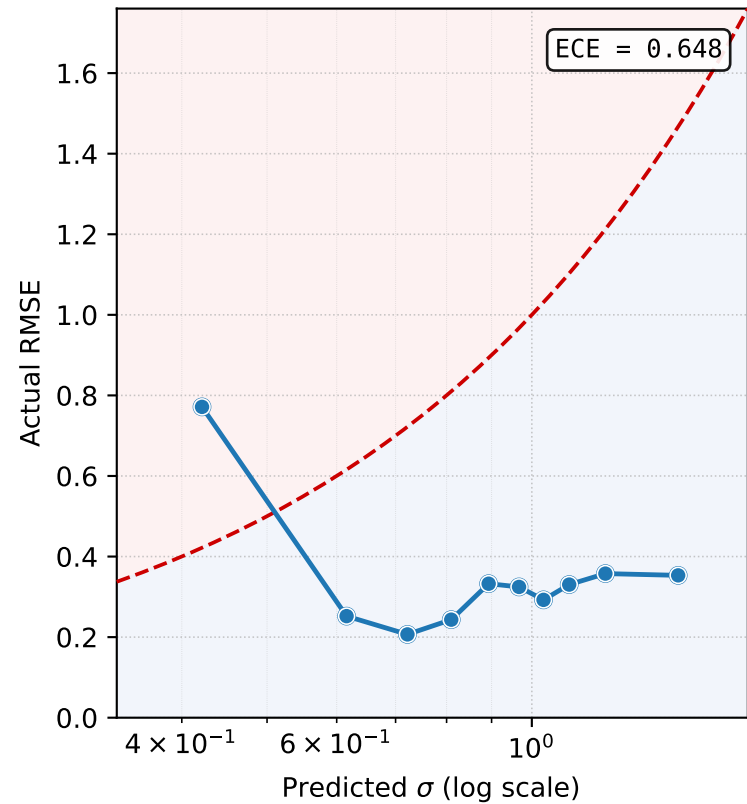
IntSeqBERT
