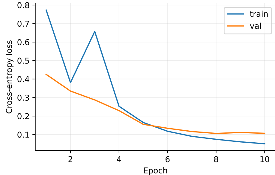
efficientnet b0
