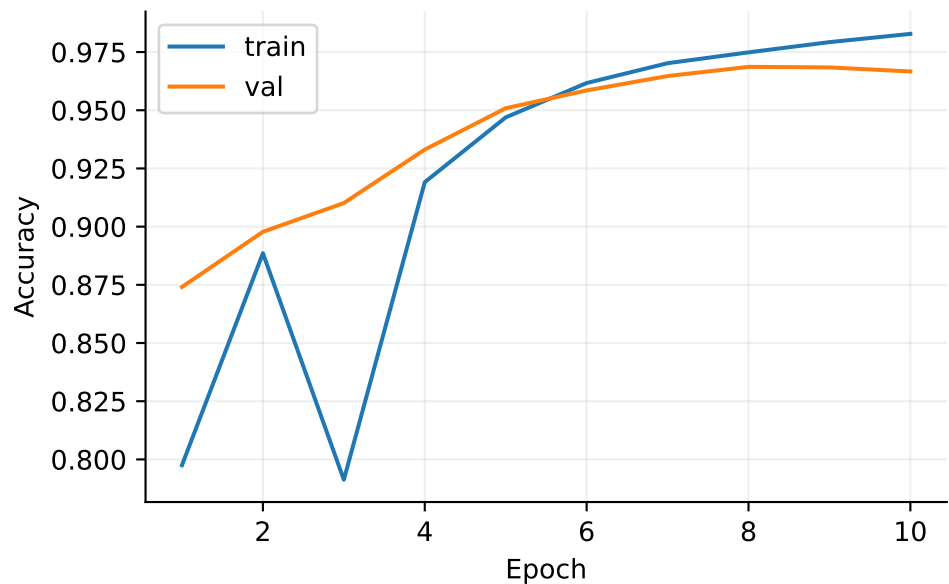
efficientnet b0
