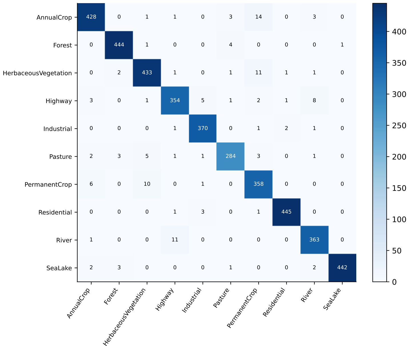
efficientnet b0
