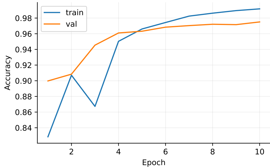
mobilenet v2
