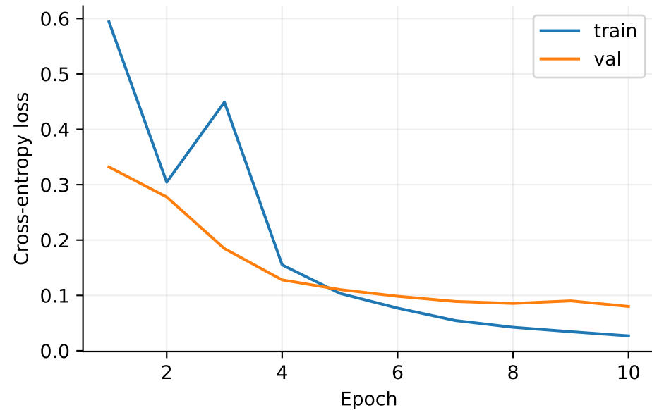
mobilenet v2
