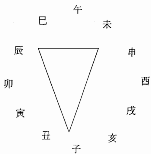
申子辰 水局
