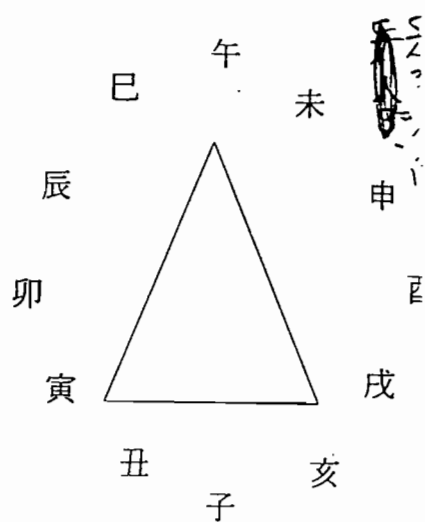
寅午戌 火局
