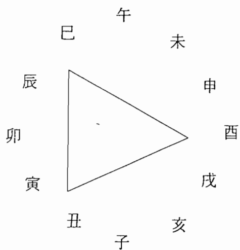
巳酉丑 金局
