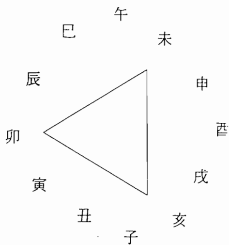
亥卯未 木局
