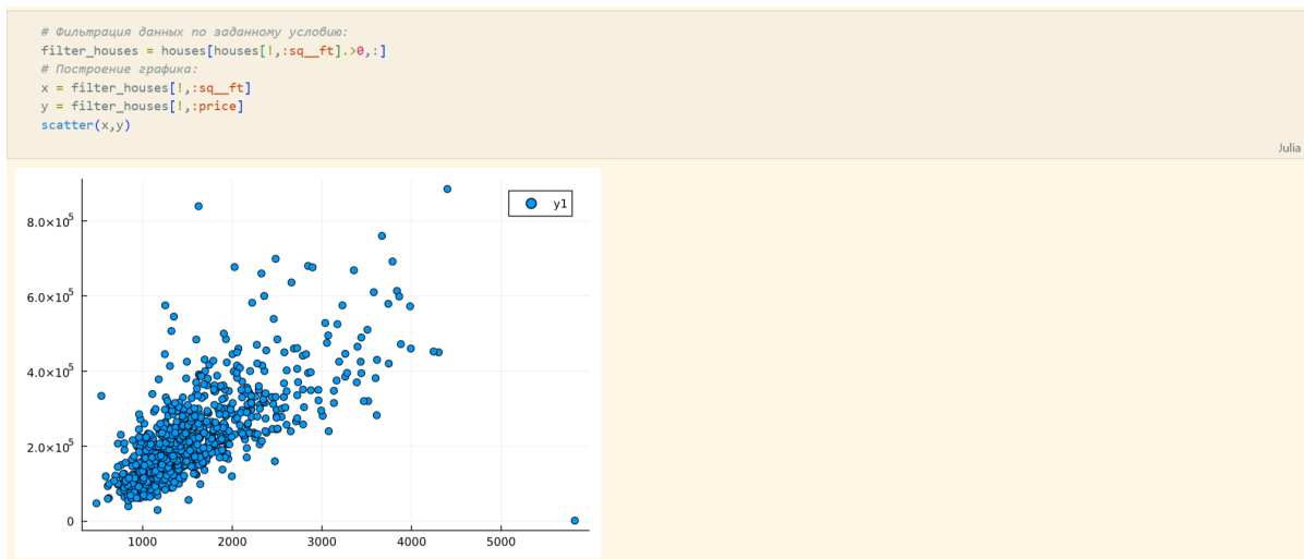
Рис. 2.25: Построение графика без “артефактов”
