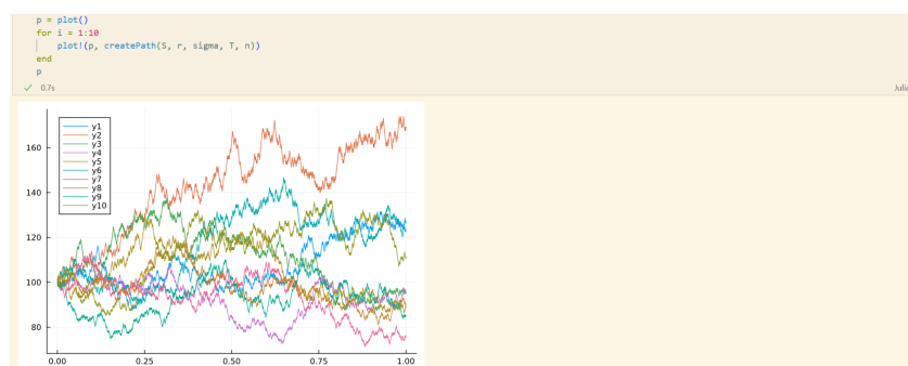
Рис. 2.46: Модель ценообразования биномиальных опционов
