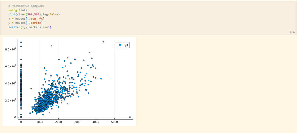
Рис. 2.24: Построение графика цен на недвижимость в зависимости от площади
