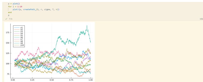
Рис. 2.48: Модель ценообразования биномиальных опционов
