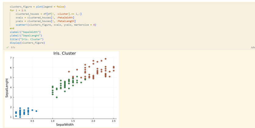
Рис. 2.39: Кластеризация
