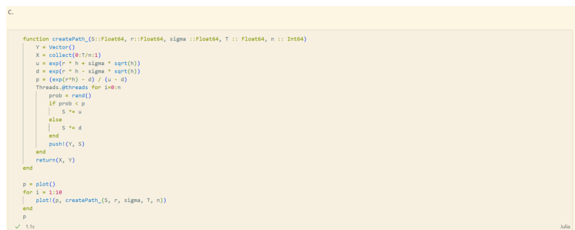
Рис. 2.47: Модель ценообразования биномиальных опционов
