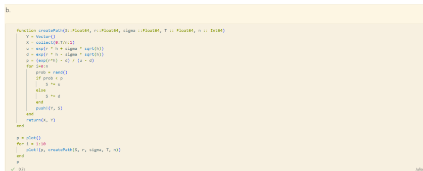
Рис. 2.45: Модель ценообразования биномиальных опционов
