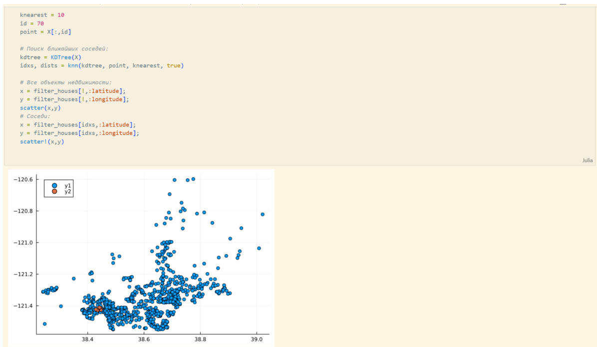
Рис. 2.30: Отображение на графике соседей выбранного объекта недвижимости
