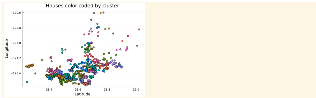
Рис. 2.28: Построение графика с кластерами разных цветов
