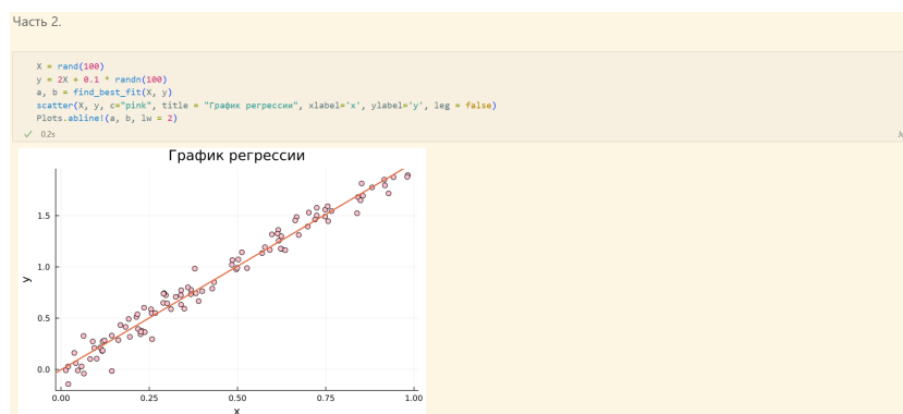
Рис. 2.42: Регрессия
