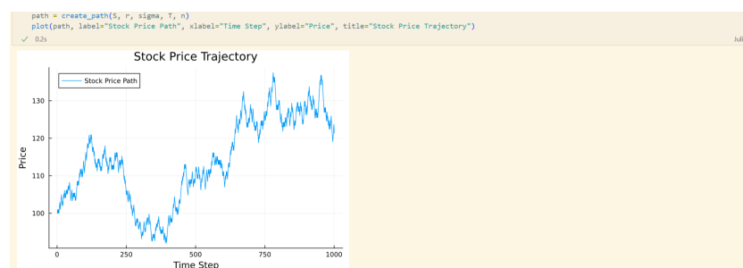
Рис. 2.44: Модель ценообразования биномиальных опционов
