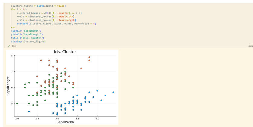
Рис. 2.38: Кластеризация
