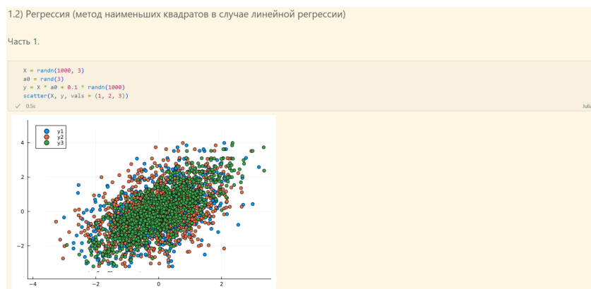
Рис. 2.40: Регрессия
