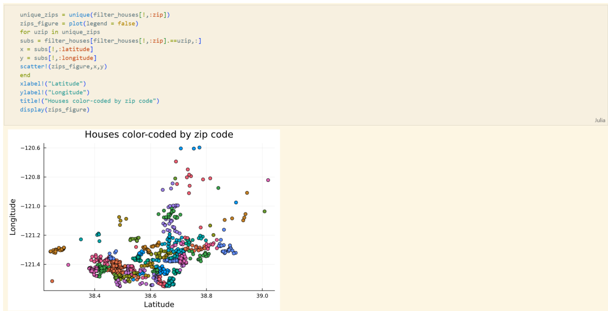
Рис. 2.29: Построение графика с кластерами разных цветов по почтовому индексу
