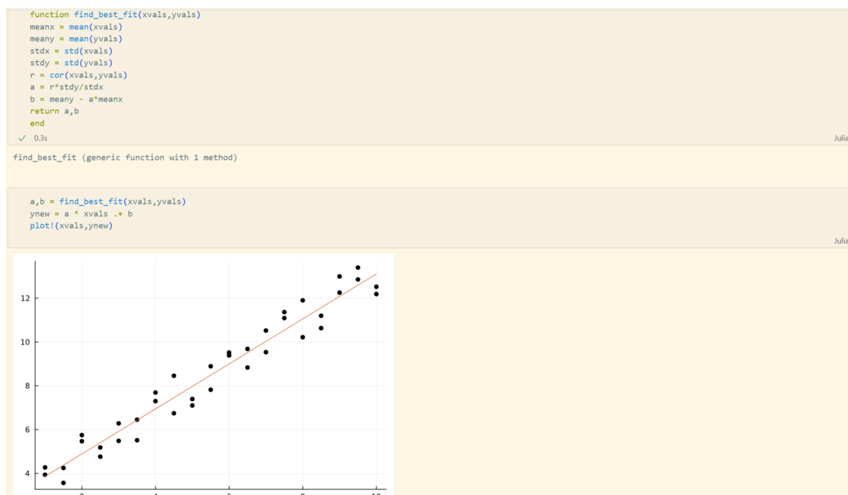
Рис. 2.34: Применение функции для построения графика
