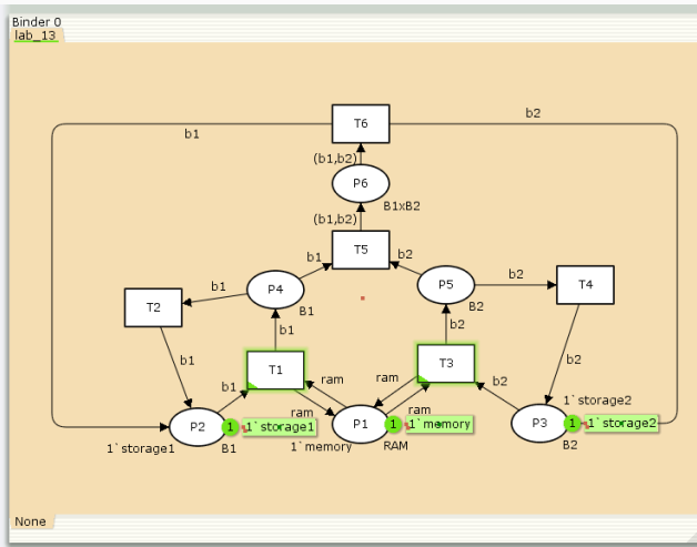
Рис. 3: Модель задачи
