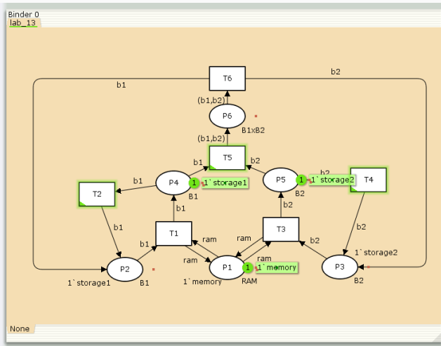
Рис. 4: Запуск модели
