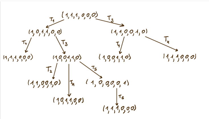
Рис. 1: Граф достижимости
