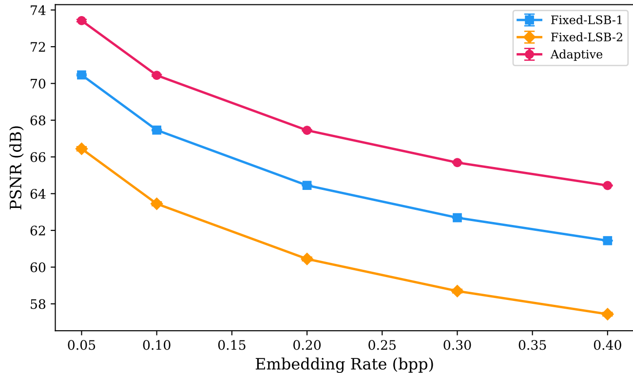
PSNR vs BPP — BOSSBase 1.01
