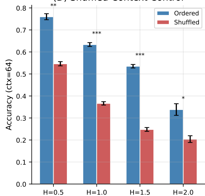
(D) Shuffled-Context Control
