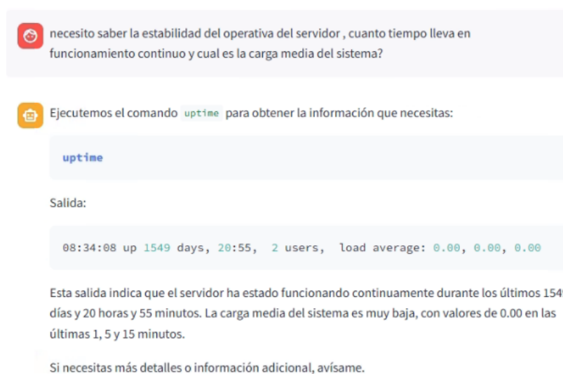
Figura 13 — Respuesta Qwen 2.5 7B (VC3): uptime ejecutado correctamente. 1549 días, 20:55. Carga 0.00.
