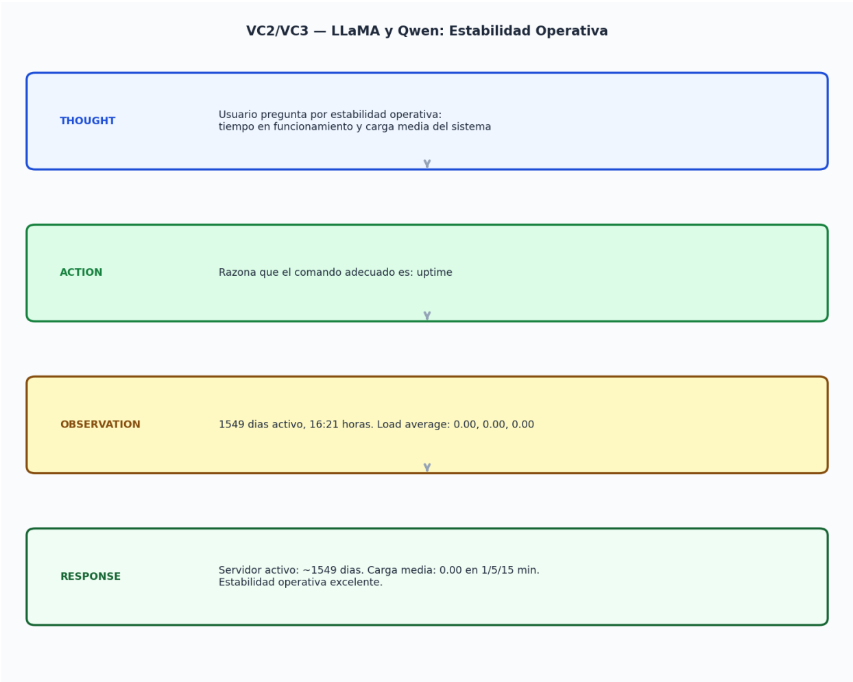
Figura 15 — Diagrama ReAct VC3 (LLaMA y Qwen): Thought → Action (uptime) → Observation → Response. Ambos modelos razonan correctamente el comando sin indicacion explicita.
