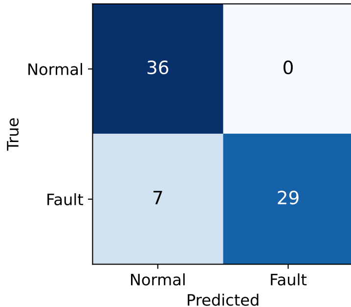
VQC (ideal)
