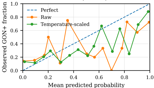
BEH (n=634)
