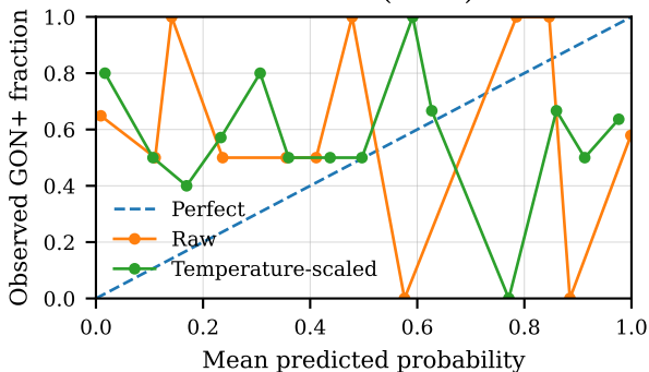
G1020 (n=1020)
