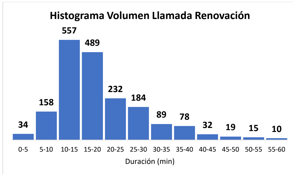
Histograma 2. Duración promedio de llamada de renovación
