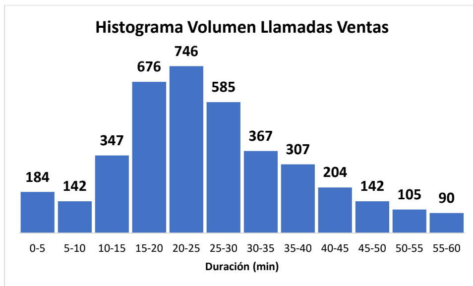
Histograma 1. Duración promedio de llamadas de venta
