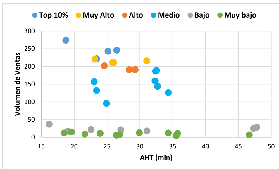
Gráfico 1. Dispersión total de ventas por agente y duración promedio de llamada
