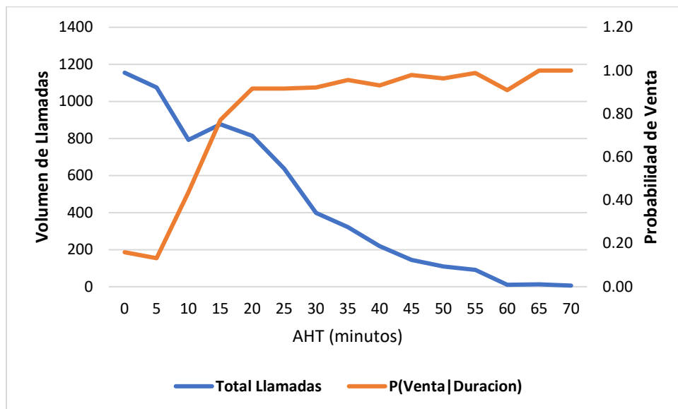
Gráfico 3. Volumen de llamadas y función densidad de probabilidad de venta
