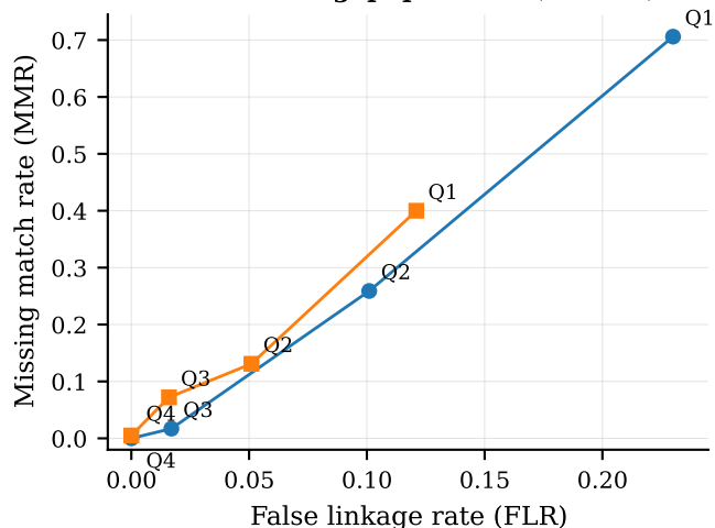
(d) Abt-Buy Discrimination-gap quartiles (Table 8)
