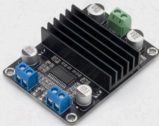
TPA3116D2 2x50W
