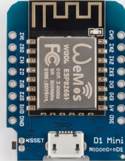
Wemos D1 Mini
