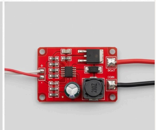
20KV Igniter Module
