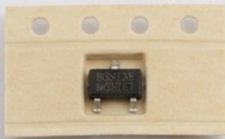
7) BSS138 MOSFET
