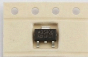
8) AO3400 MOSFET
