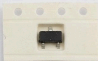
5) MMBT3906 PNP
