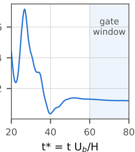
(b) Drag, C_D = 2F_x
