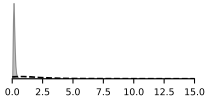
F. \phi (overdispersion)
