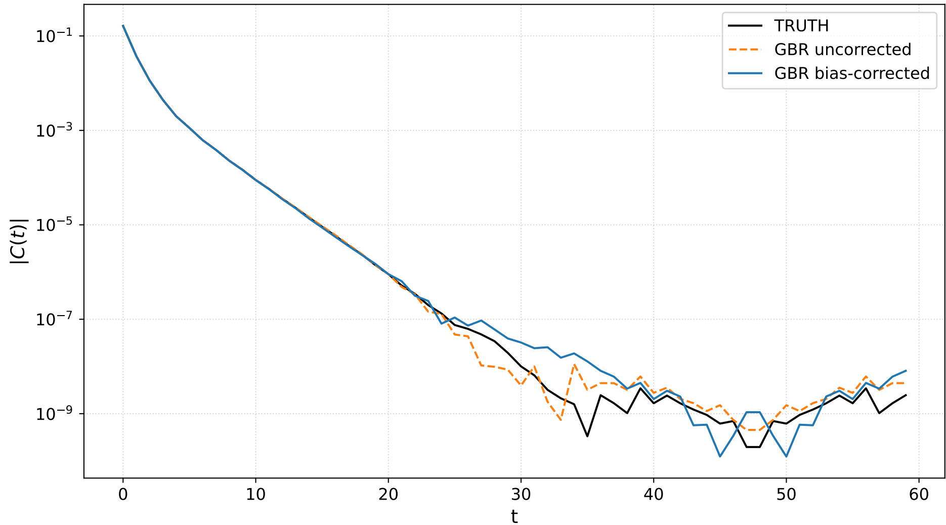
Bias correction effect (GBR)
