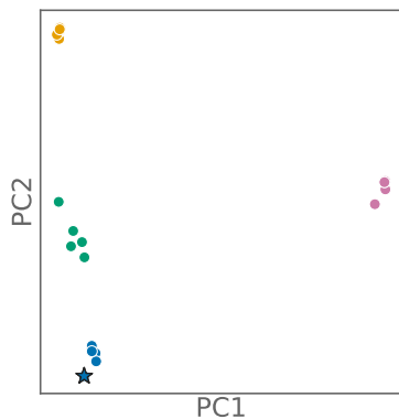
standard PCA min R^2 = 0.228
