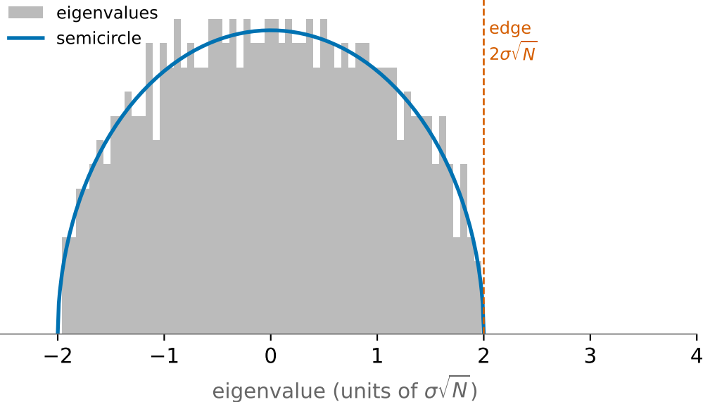
pure noise
