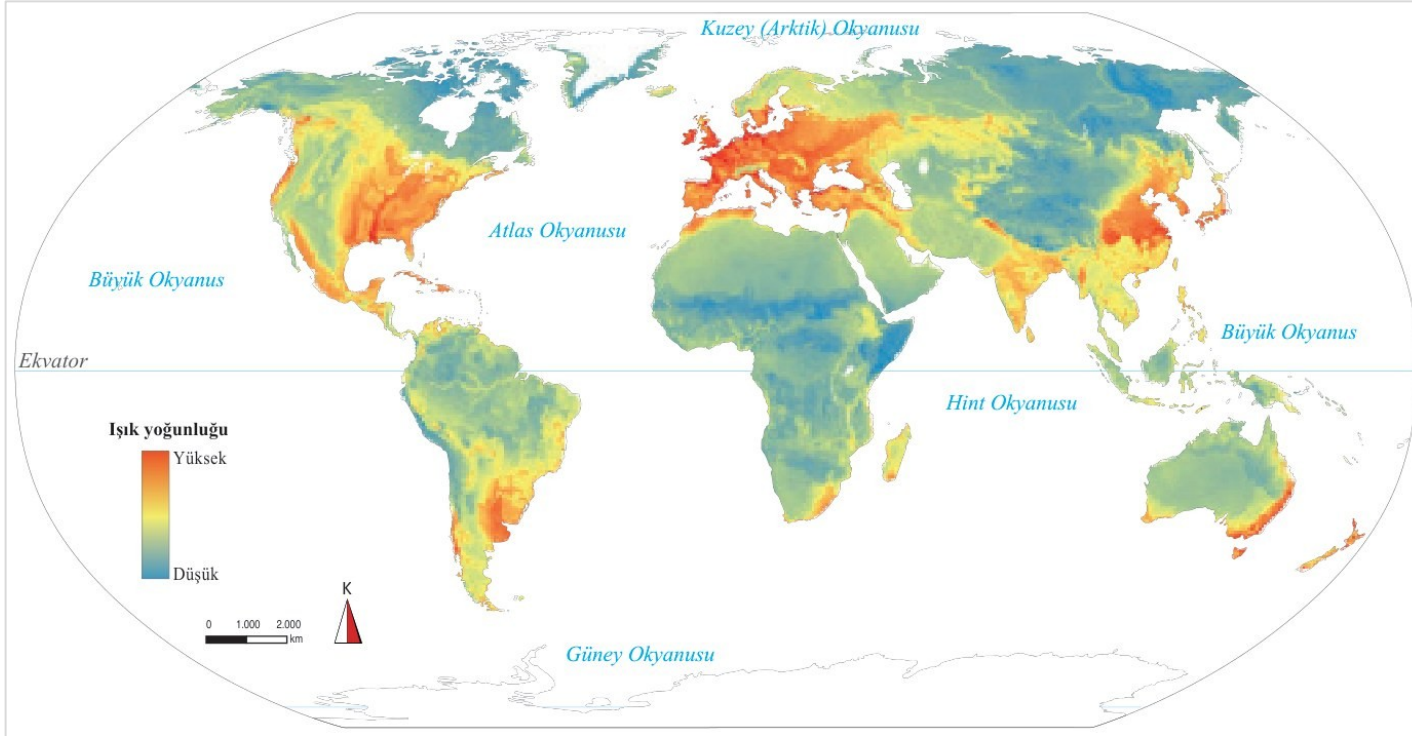
Kitap s. 173: gece ışıklarının küresel dağılımı
