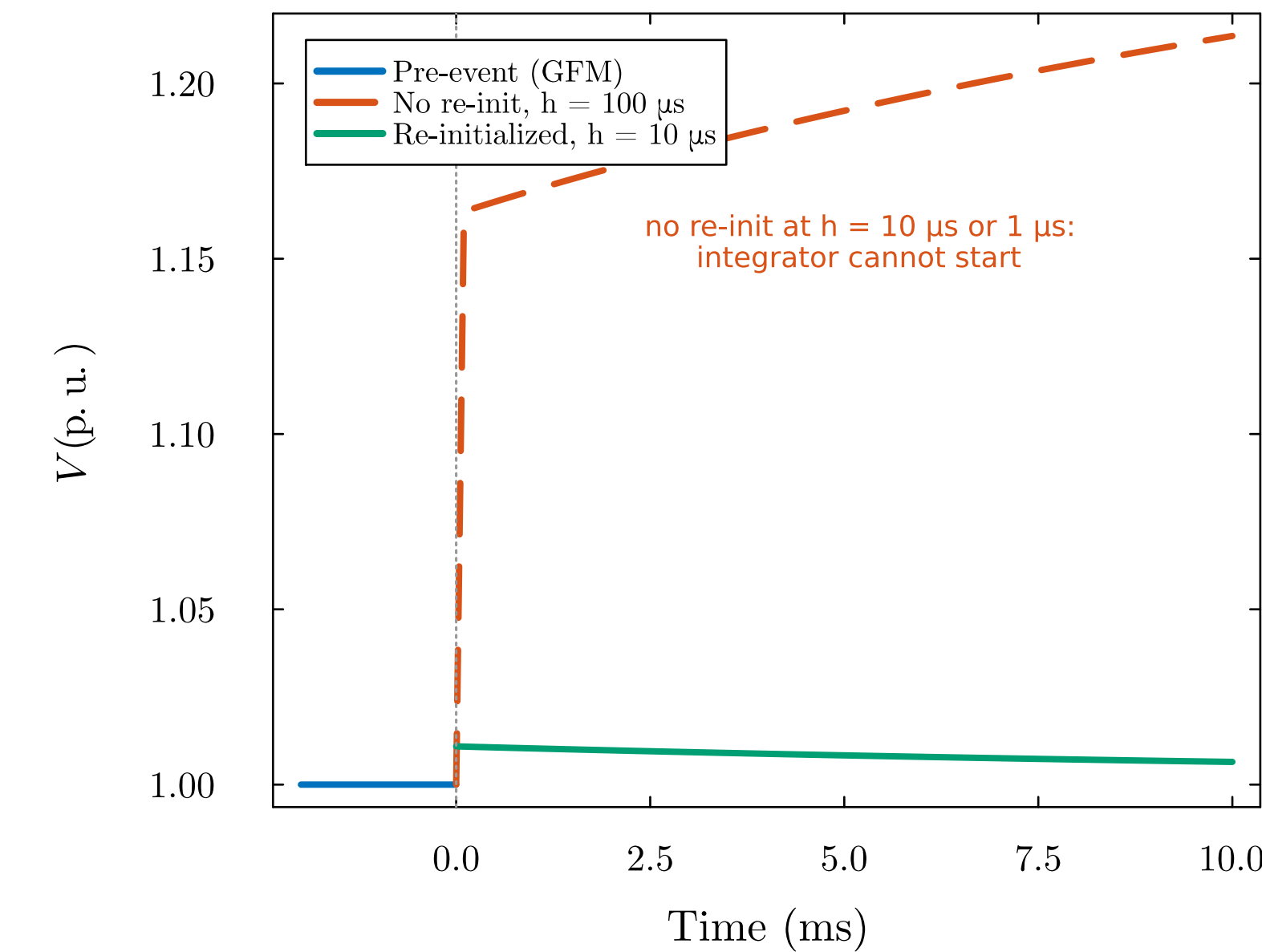
(d) PCC voltage
