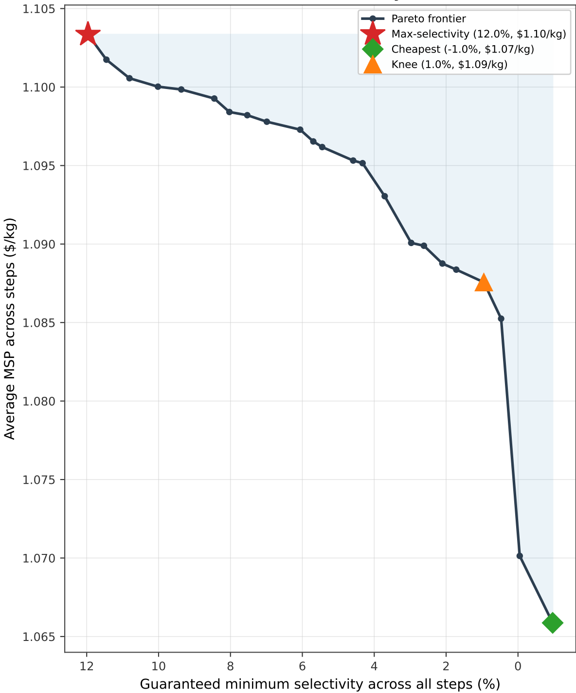
Pareto frontier: selectivity vs cost
