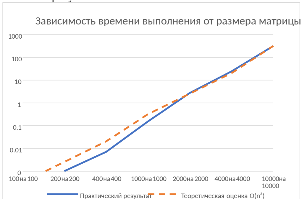
Рис.2 – график зависимости времени выполнения программы от размера матриц.
