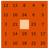
24-puzzle (scale)
