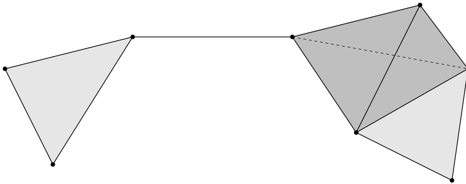
Rysunek 2.2: kompleks symplecjajny
