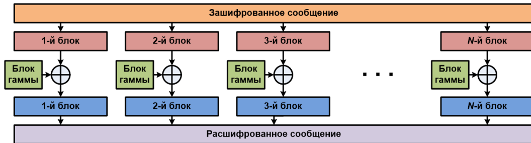
Рисунок 2: Дешифровка
