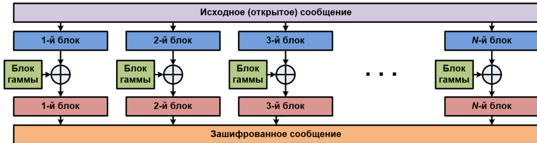
Рисунок 1: Шифрование
