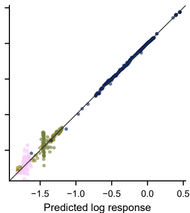
(d) Lagging leaky SD=0.174
