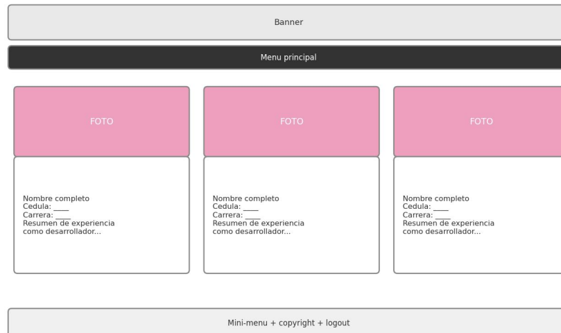
Figura 5. Wireframe de sobre_nosotros.jsp.
