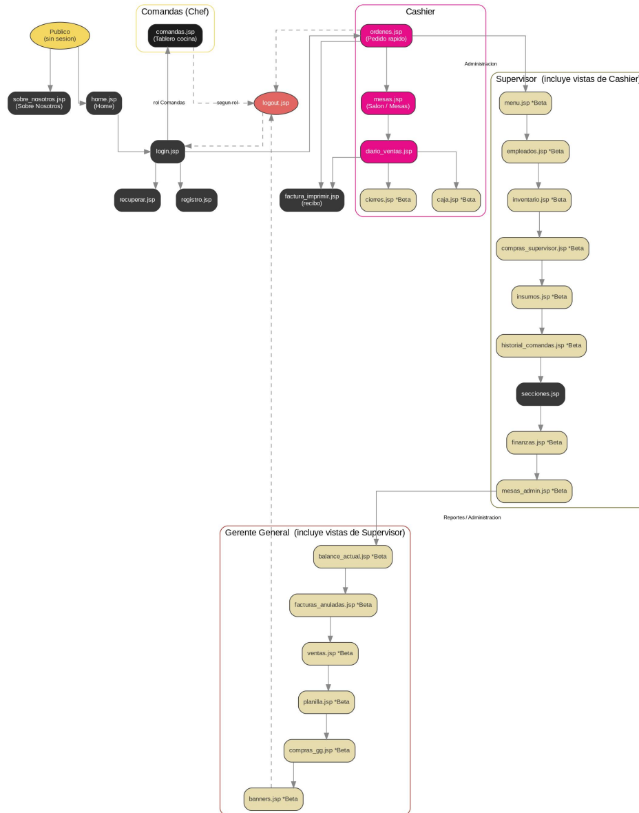
Figura 1. Mapa de navegacion del sitio MiPedido, agrupado por rol de usuario.
