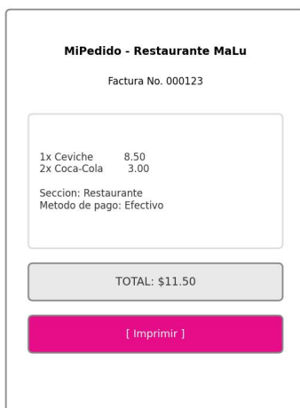
Figura 11. Wireframe de referencia para el recibo/factura del cliente. En la implementación final el detalle de la factura se muestra dentro de pages/ventas.jsp (acción verFactura ), sin una página .jsp separada de impresión.
