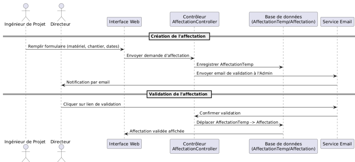
FIGURE 4 : DIAGRAMME DE SEQUENCE AFFECTATION
