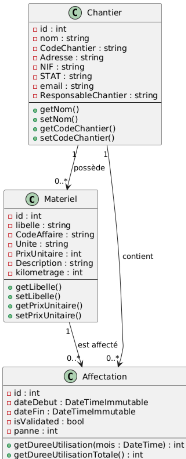
FIGURE 3 : DIAGRAMME DE CLASSE
