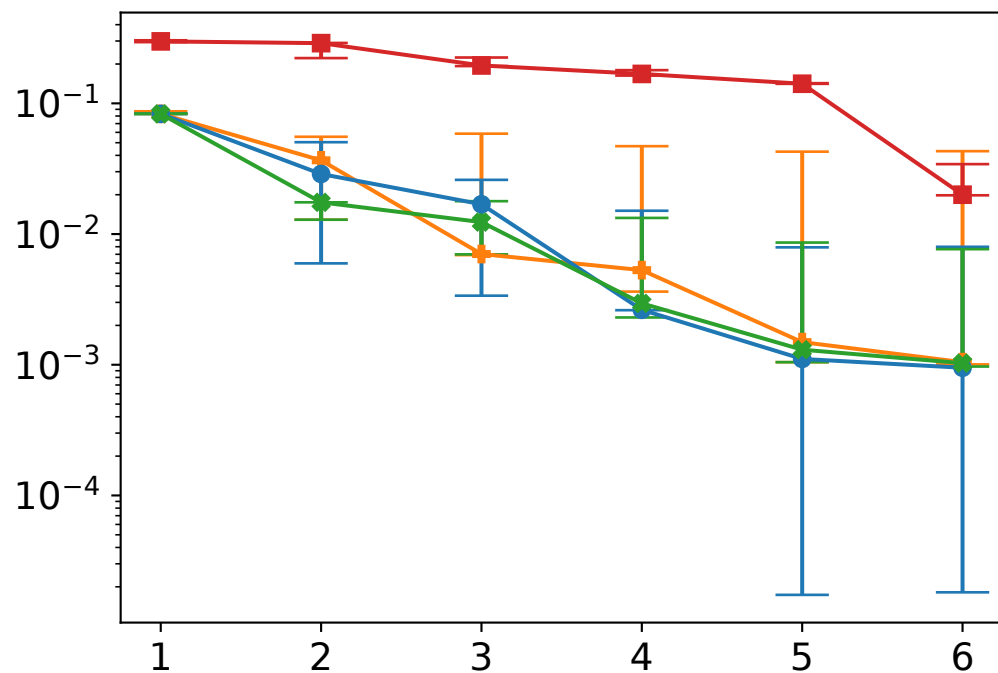
Train MSE
