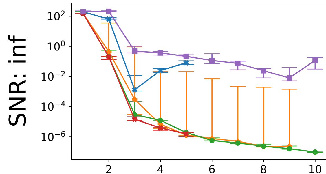
Train MSE
