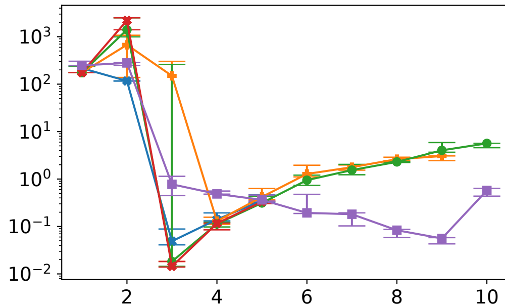
Test MSE
