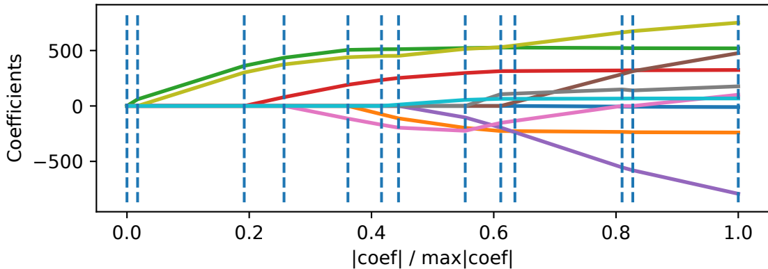
LASSO Path
