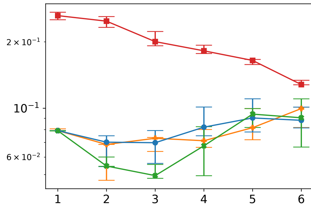
Test MSE
