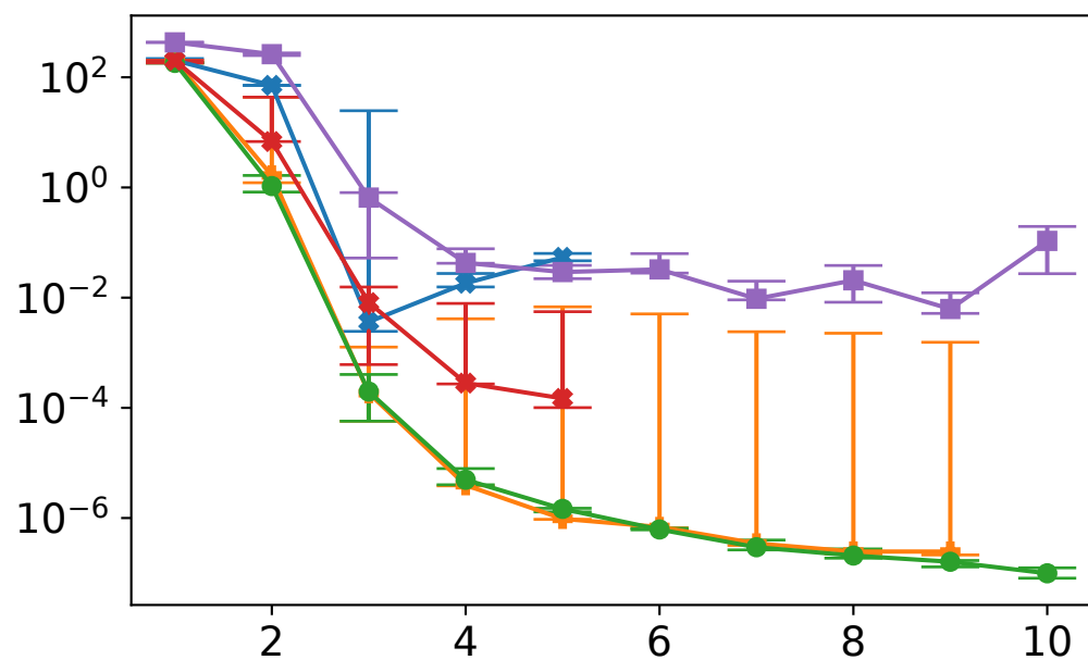
SNR: 2
