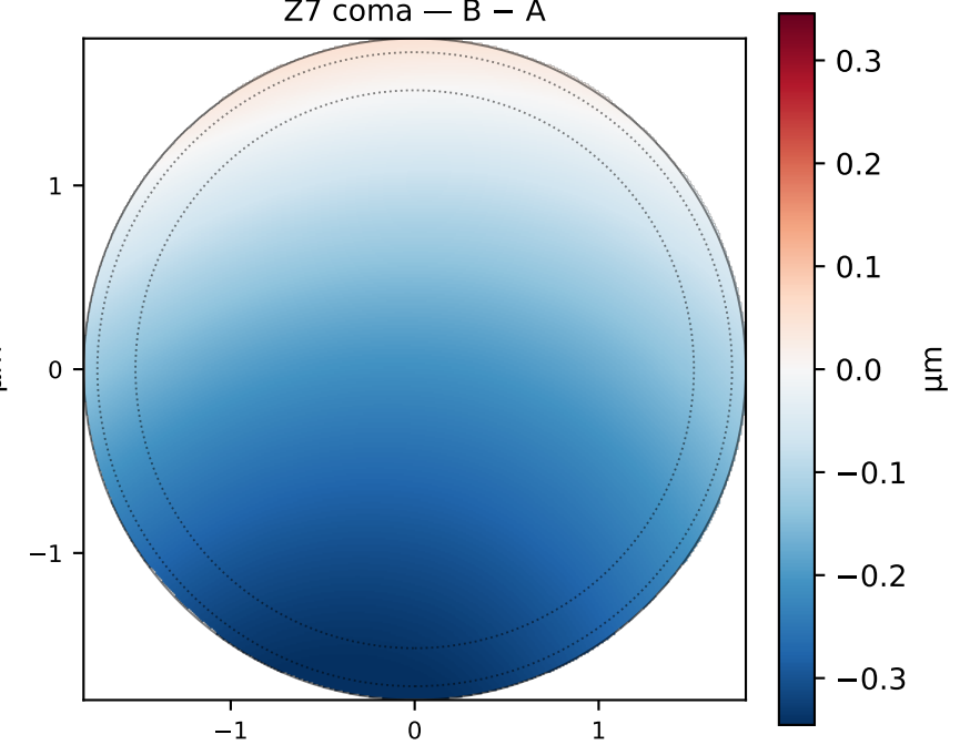
Z7 coma — B - A
