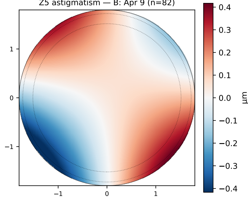
Z5 astigmatism — B: Apr 9 (n=82)
