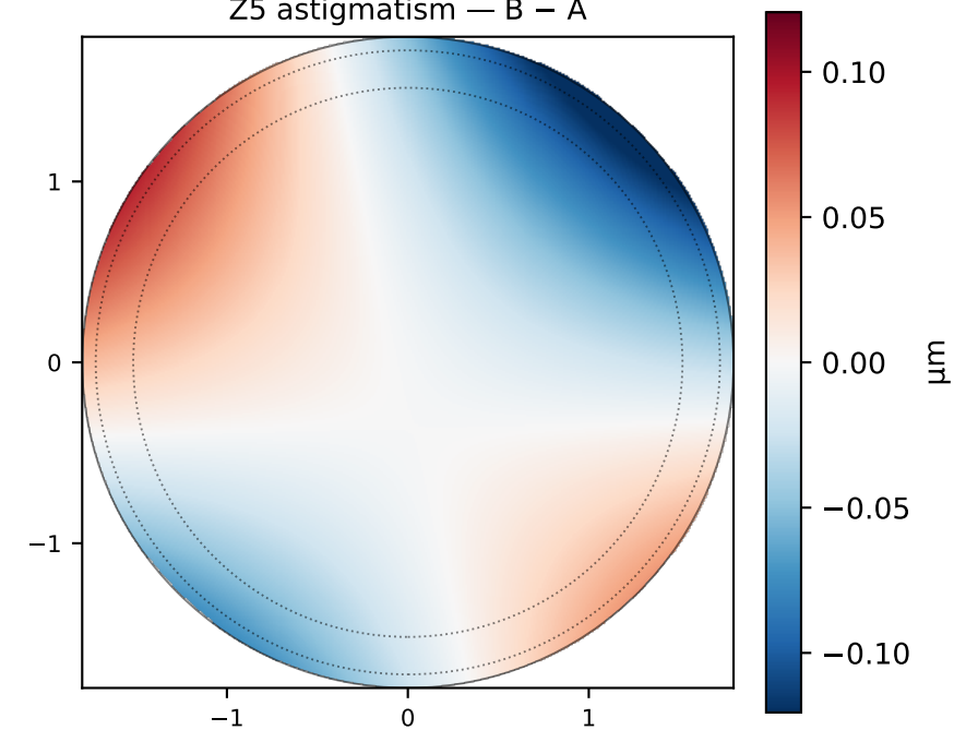
Z5 astigmatism — B - A
