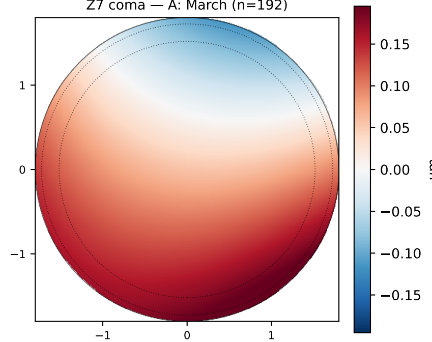
Z7 coma — A: March (n=192)
