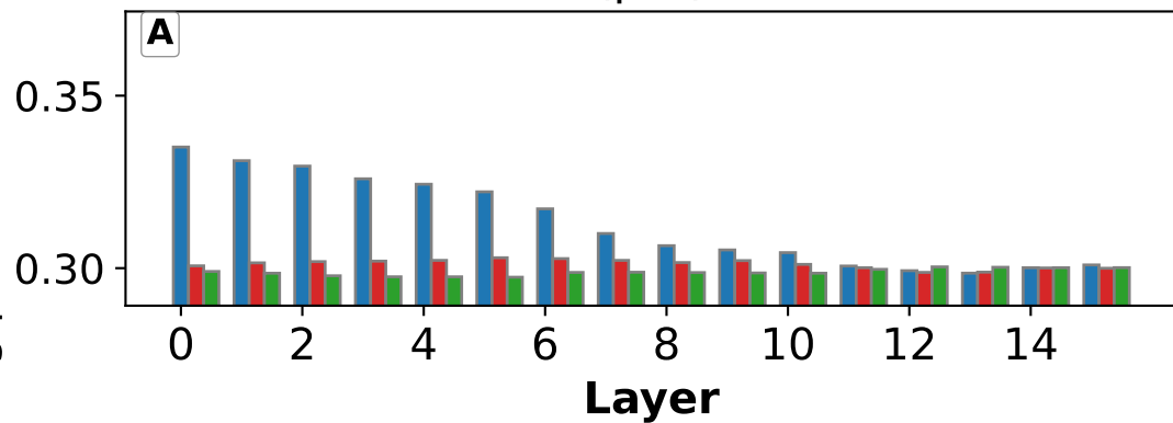
OLMo-2-0425-1B (pre)
