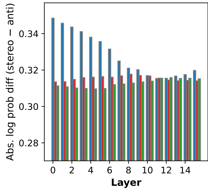
(d) Gender bias effect of different words (OLMo-2-0425-1B)
