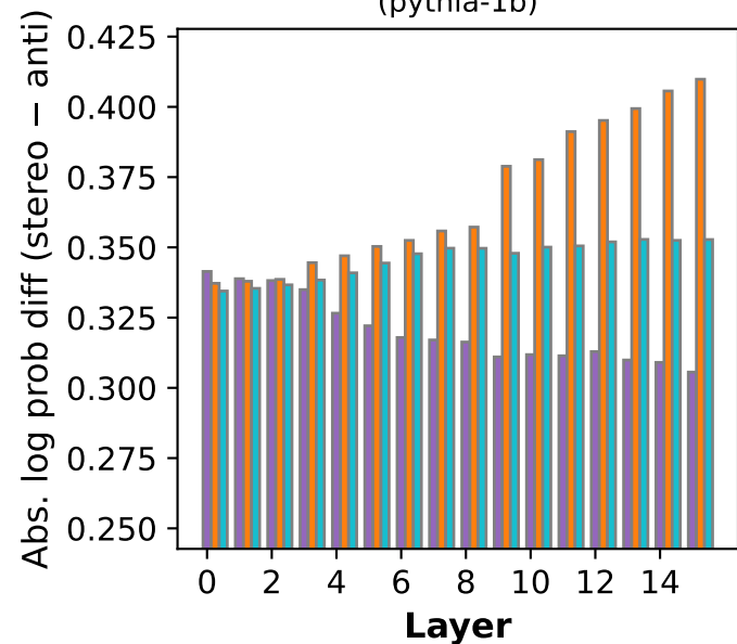
(d) Gender bias effect of different words (pythia-1b)
