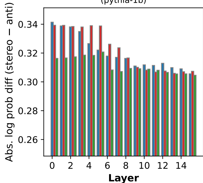
(d) Gender bias effect of different words (pythia-1b)
