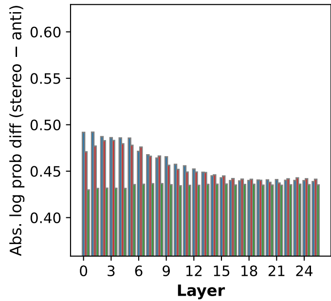
(d) Gender bias effect of different words (gemma-3-1b-pt)
