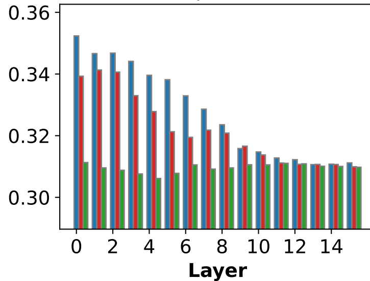
(b) Llama-3.2-1B-Instruct (post)
