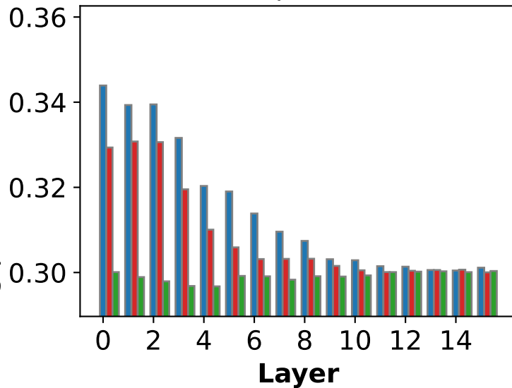
(a) Llama-3.2-1B (pre)
