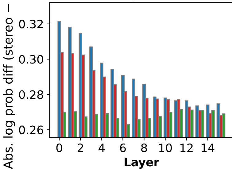
(a) Llama-3.2-1B (pre)
